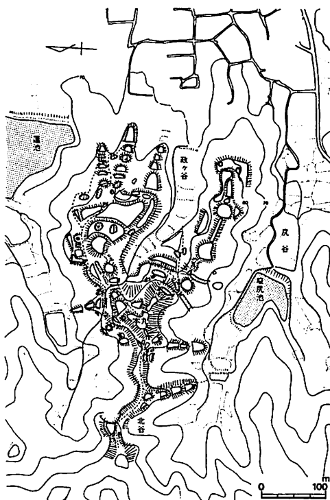
第182図 稲屋妻城跡平面図(土橋誠「府下遺跡紹介26. 稲八間城跡」〔『京都府埋蔵文化財情報』第15号掲載, 京都, 昭和60年〕より転載)
