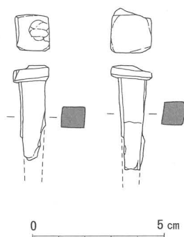
Fig.11 鉄釘実測図
