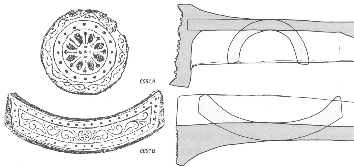
Fig. 6 軒瓦6091A-6691B 1:4
