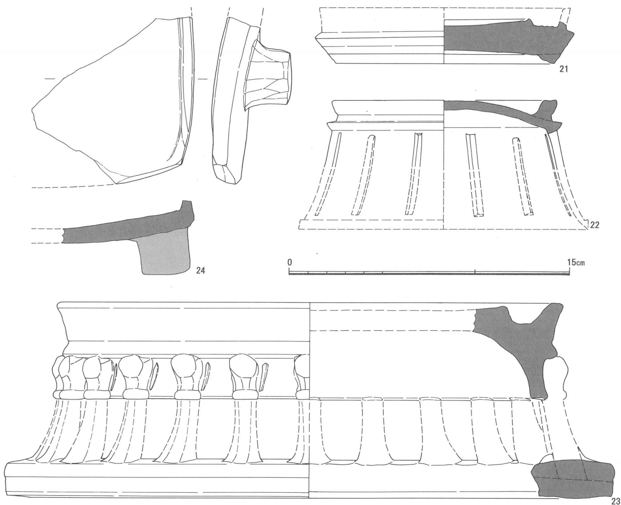
Fig.10 陶硯実測図 1:2
