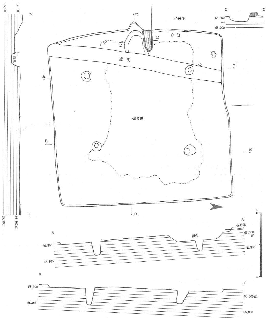
第98図 48号住居跡実測図
