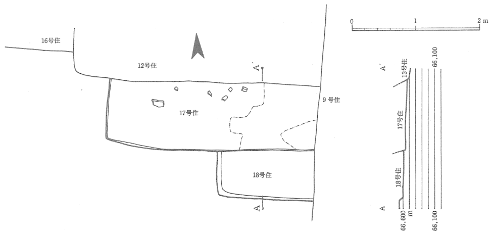
第64図 17・18号住居跡実測図
