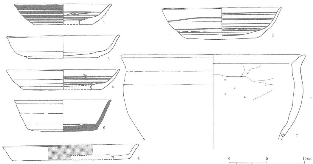
第51図 7号住居跡内出土土器実測図
