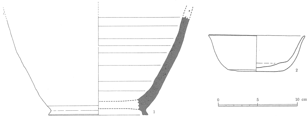
第80図 30号住居跡内出土土器実測図
