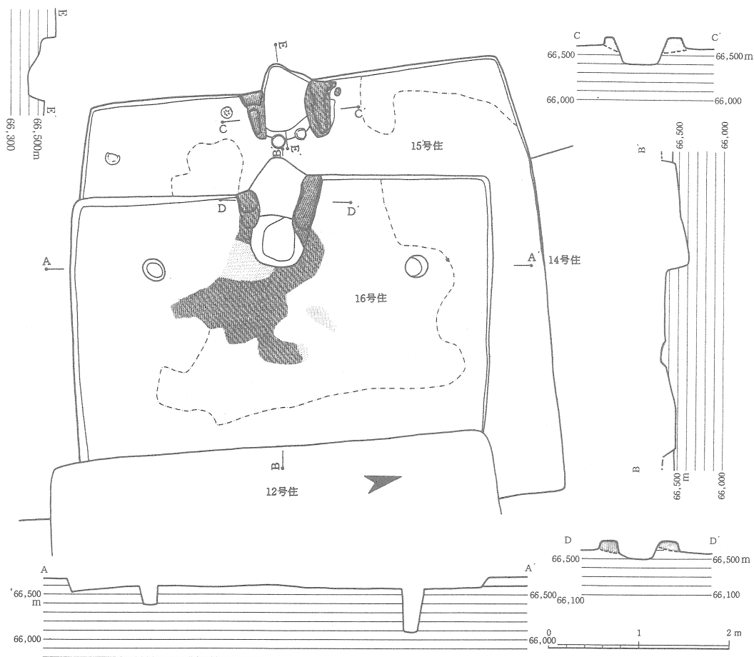
第61図 15号・16号住居跡実測図
