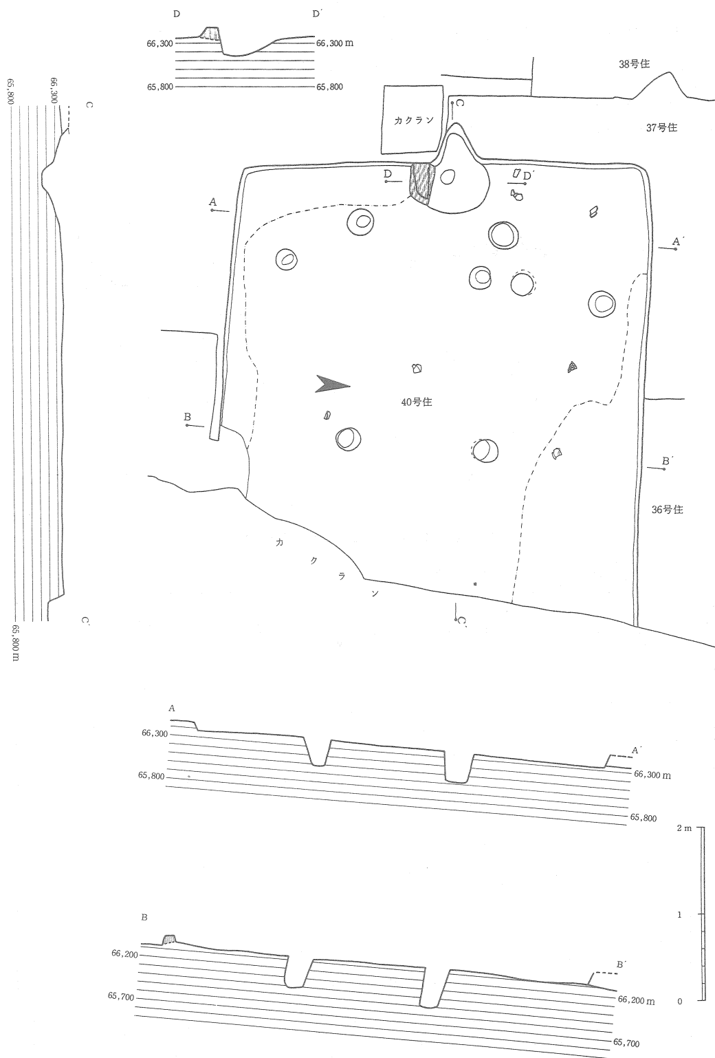
第89図 40号住居跡実測図
