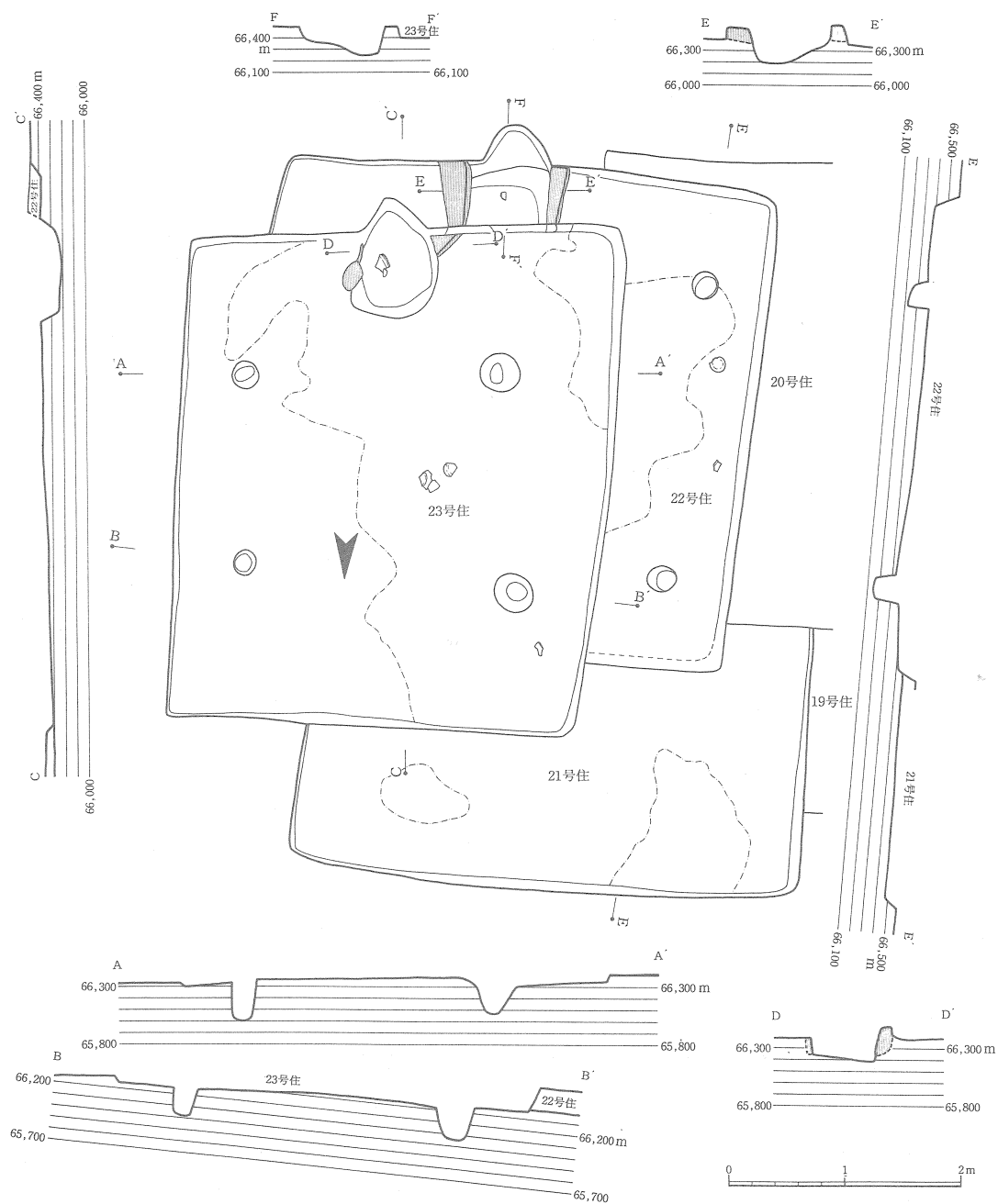
第67図 21号・22号・23号住居跡実測図
