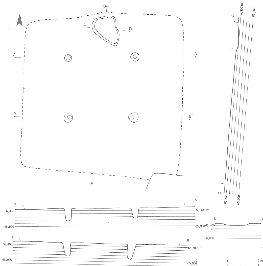
第84図 33号住居跡実測図
