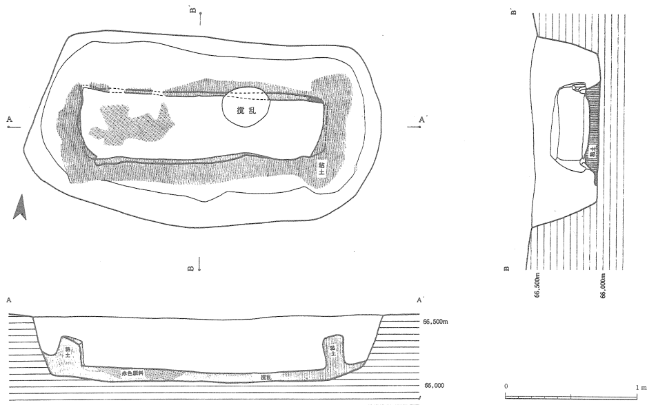
第36図 9号方形周溝墓主体部実測図
