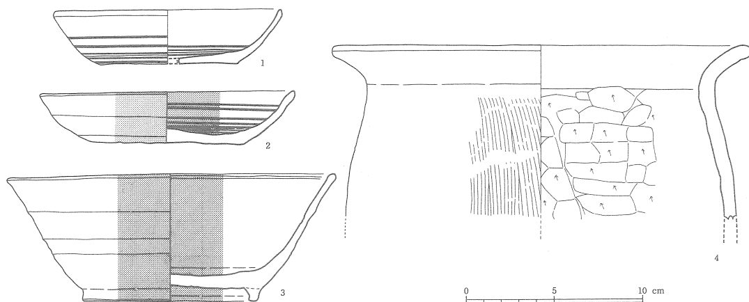
第70図 23号住居跡内出土土器実測図
