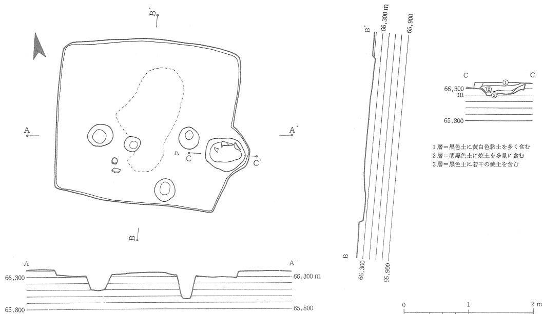
第50図 7号住居跡実測図
