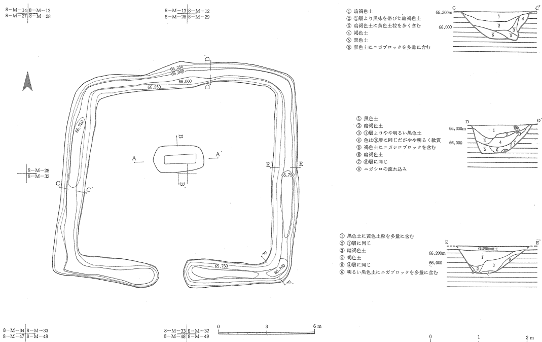
第31図 7号方形周溝墓測量図及び周溝土層判断図
