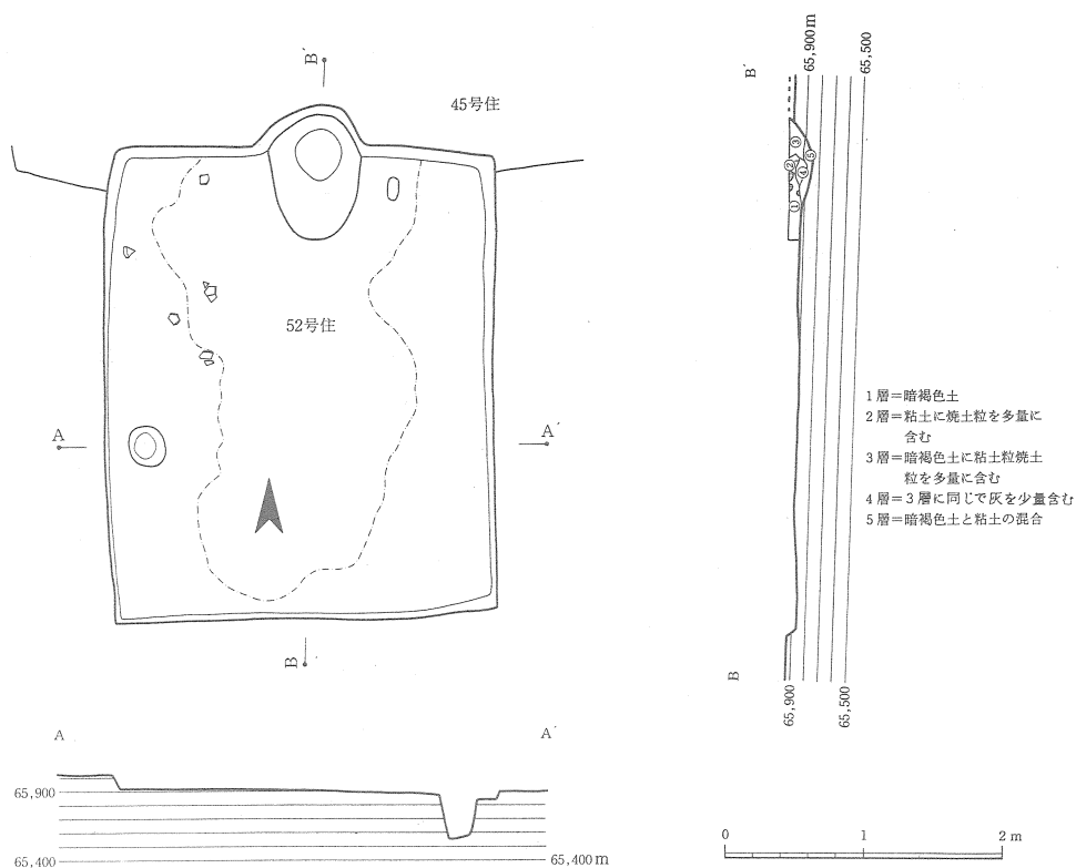
第104図 52号住居跡実測図
