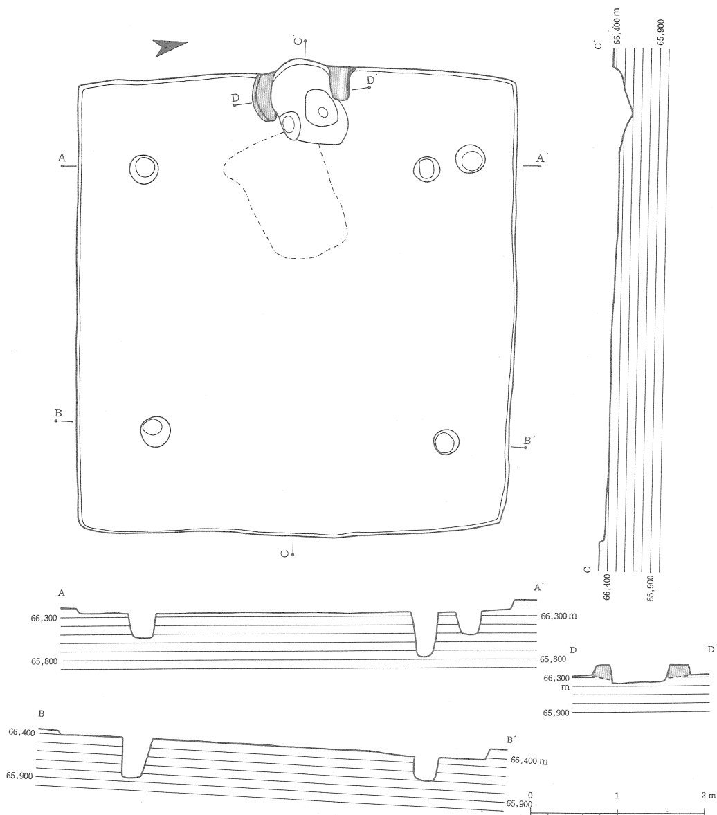
第103図 51号住居跡実測図
