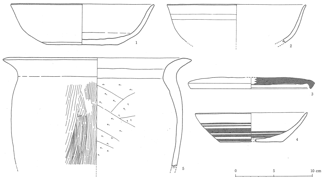
第99図 48号住居跡内出土土器実測図
