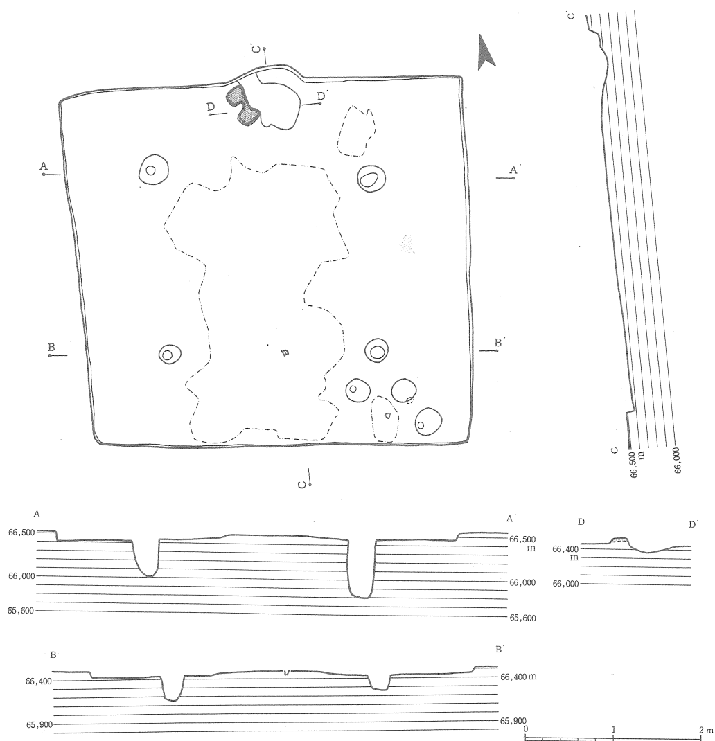
第71図 24号住居跡実測図
