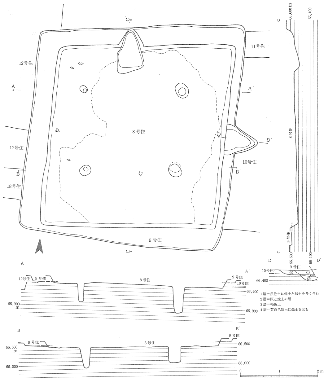
第52図 8号・9号住居跡実測図
