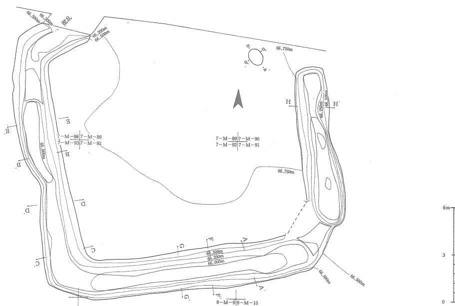
第22図 5号方形周溝墓測量図
