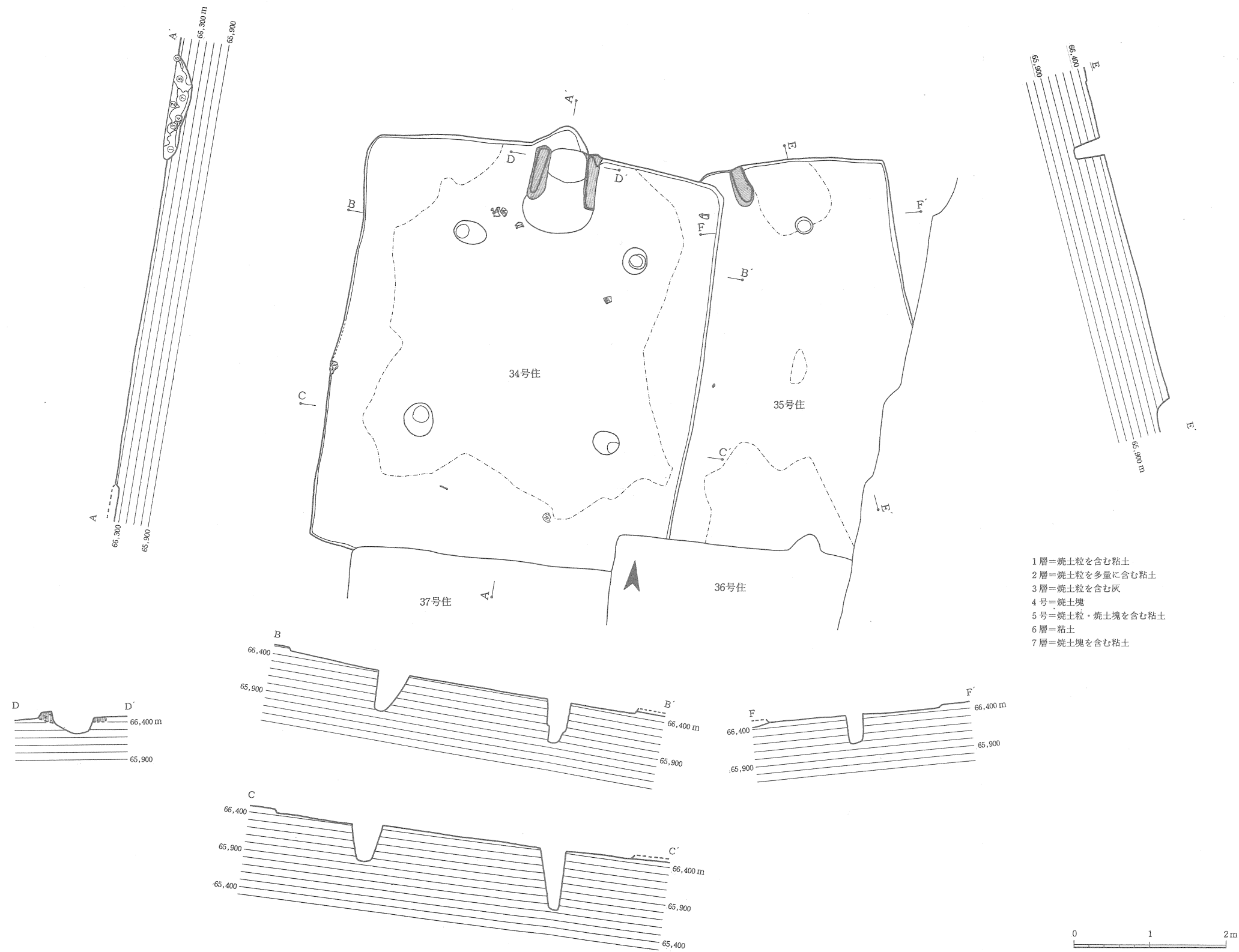
第85図 34号・35号住居跡実測図
