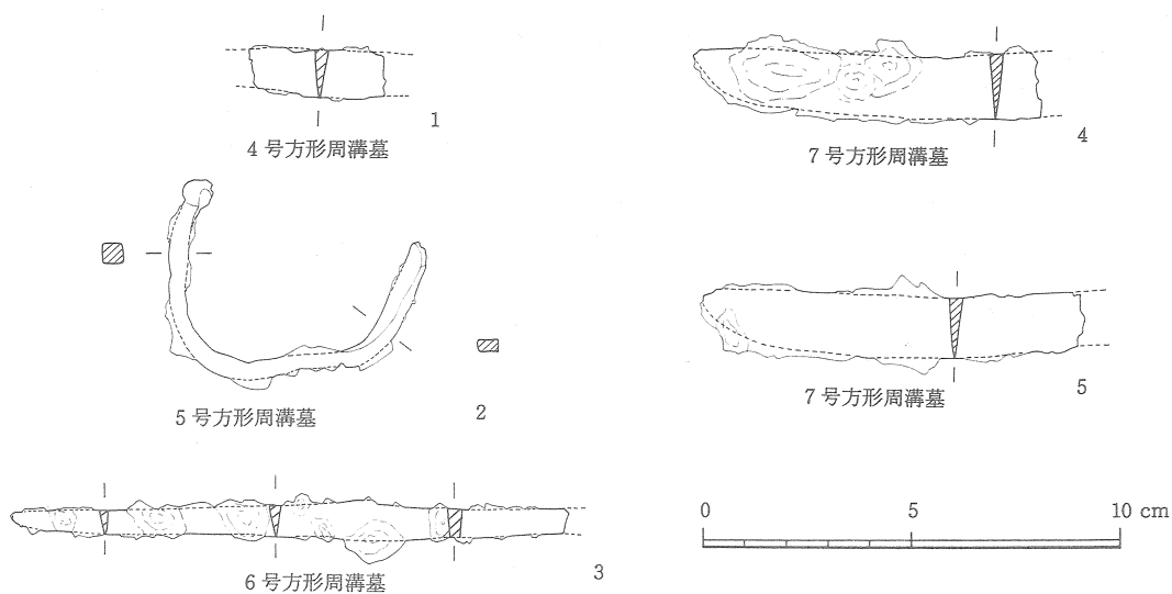
第41図 方形周溝墓内出土鉄器実測図
