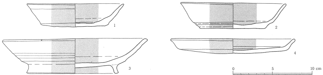
第62図 15号住居跡内出土土器実測図
