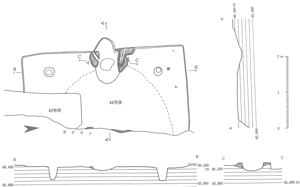
第91図 42号住居跡実測図
