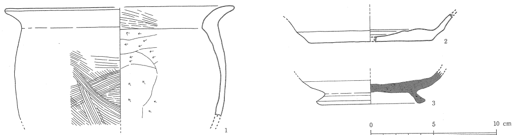
第76図 27号住居跡内出土土器実測図
