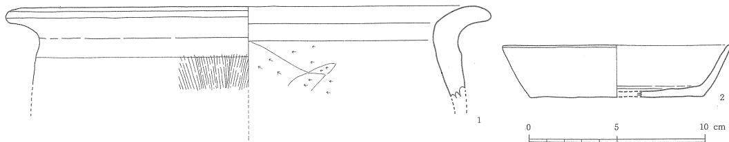
第111図 55号住居跡内出土土器実測図
