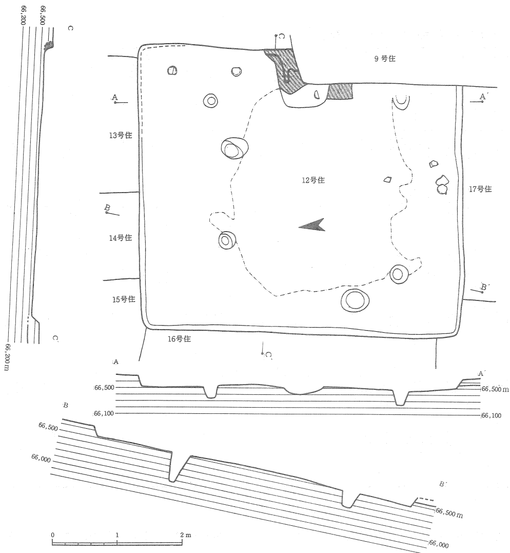
第56図 12号住居跡実測図
