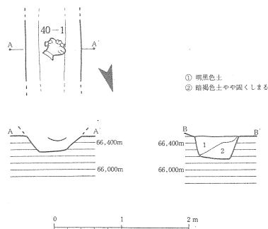
第39図 11号方形周溝墓測量図及び周溝内遺物出土状態実測図
