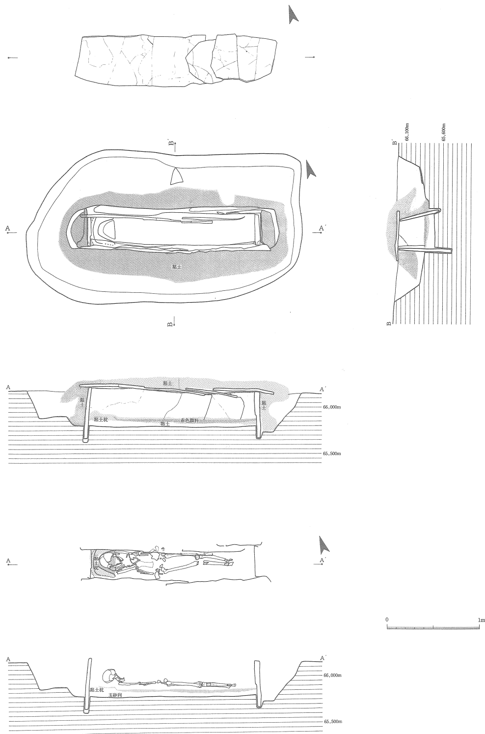
第19図 3号方形周溝墓主体部石棺及び石棺内人骨出土状態実測図
