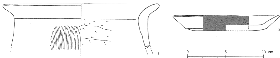
第74図 26号住居跡内出土土器実測図
