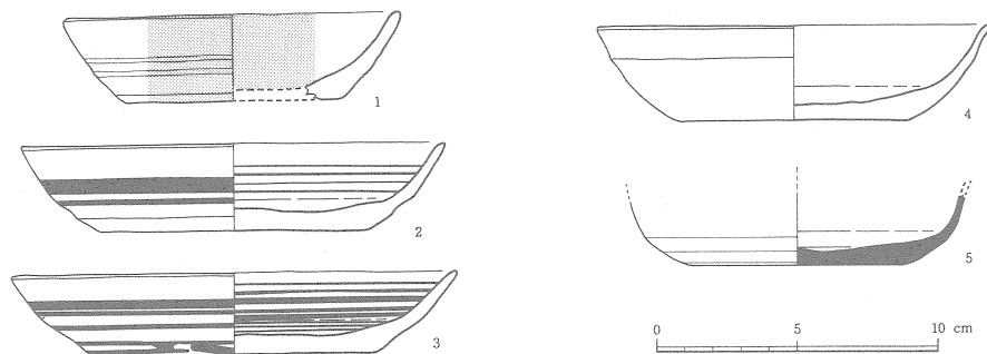
第82図 31号住居跡内出土土器実測図
