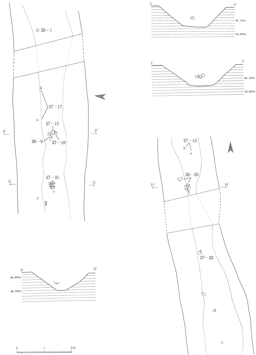
第24图 5号方形周溝墓周溝内遺物出土状态实测图
