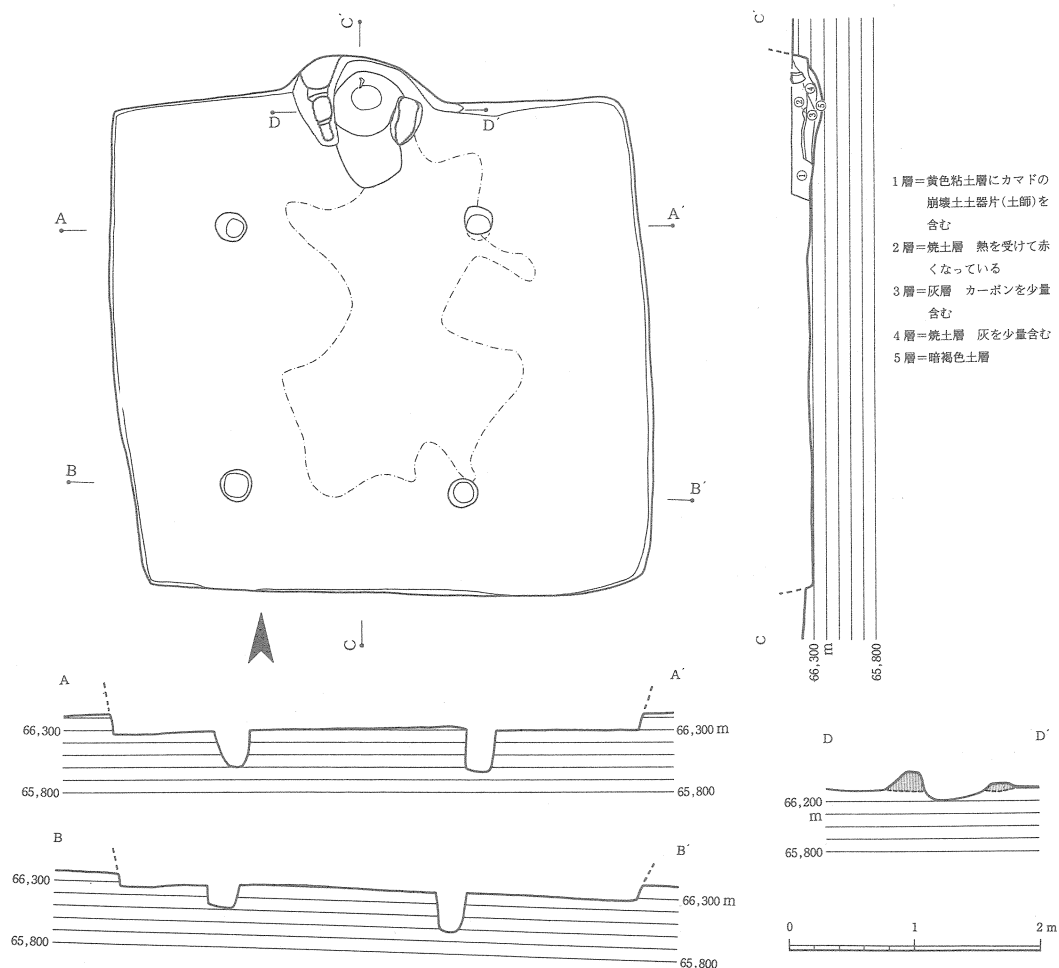
第95図 46号住居跡実測図
