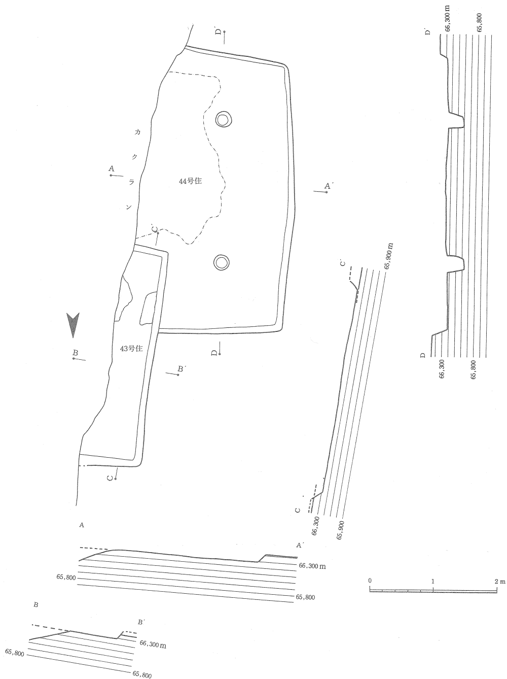
第93図 43号・44号住居跡実測図
