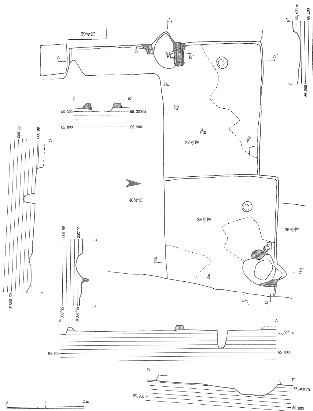
第86図 36号・37号住居跡実測図
