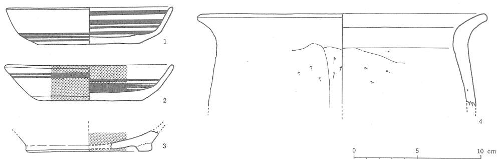
第66図 20号住居跡内出土土器実測図
