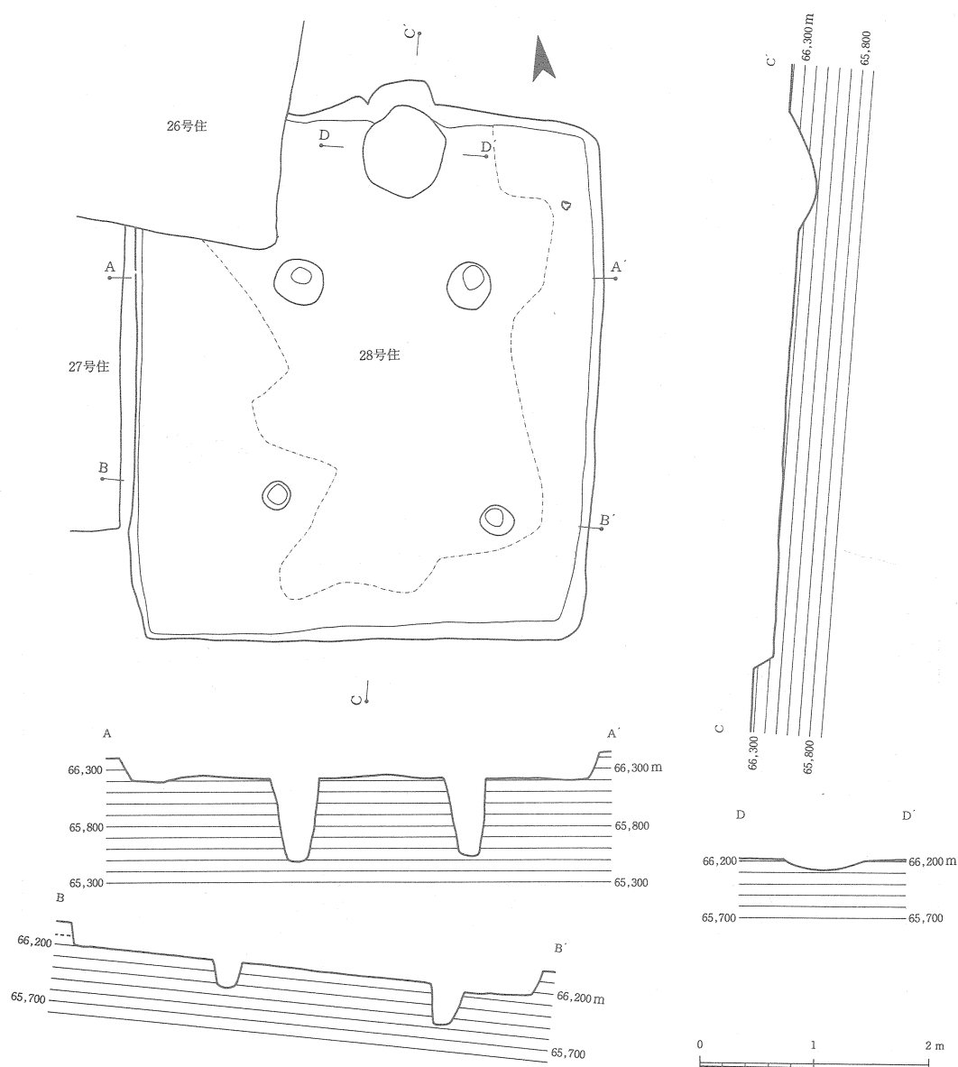
第77図 28号住居跡実測図
