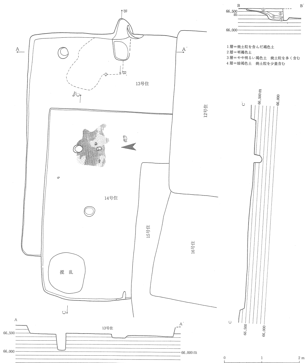
第58図 13号・14号住居跡実測図
