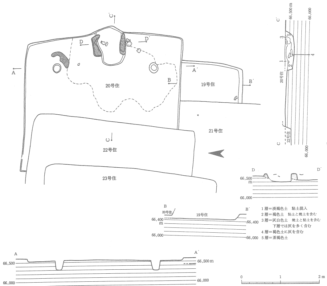
第65図 19号・20号住居跡実測図
