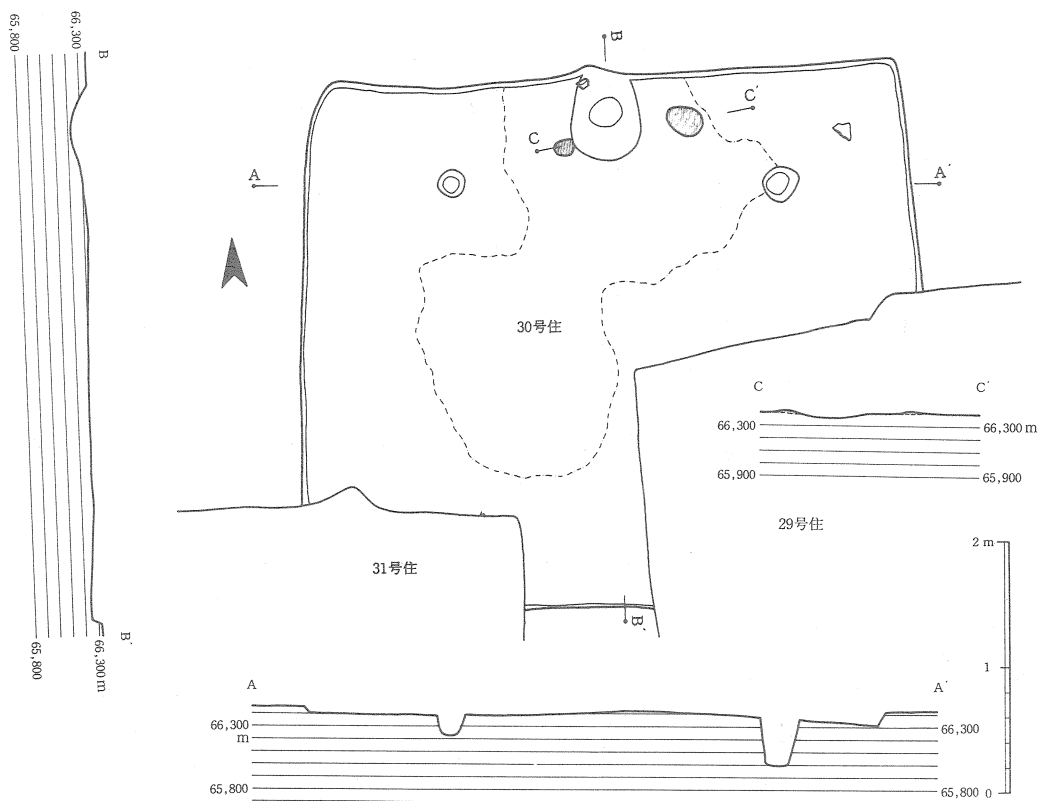
第79図 30号住居跡実測図
