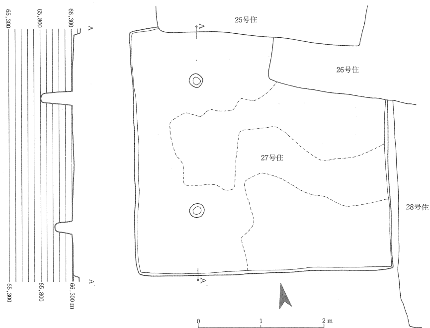
第75図 27号住居跡実測図
