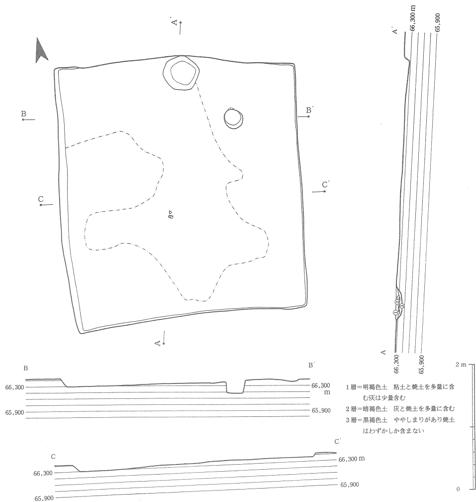
第110図 55号住居跡実測図
