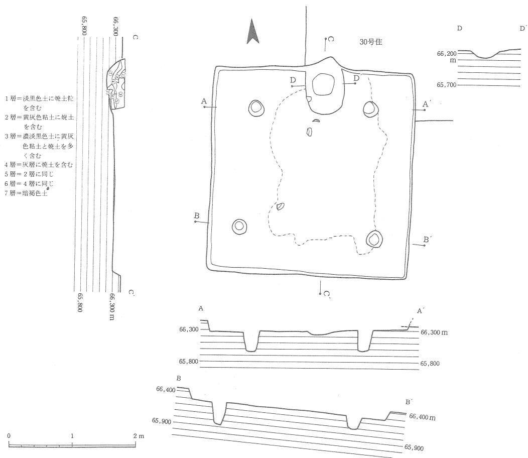
第81図 31号住居跡実測図
