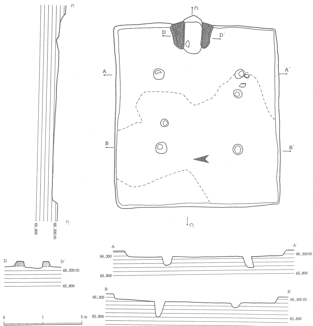
第106図 53号住居跡実測図
