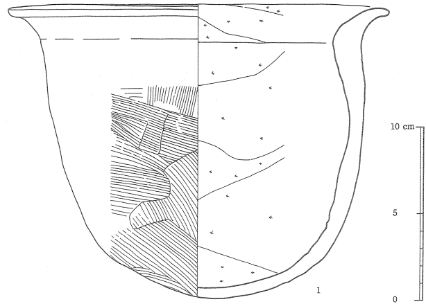
第101図 49号住居跡カマド内出土土器実測図
