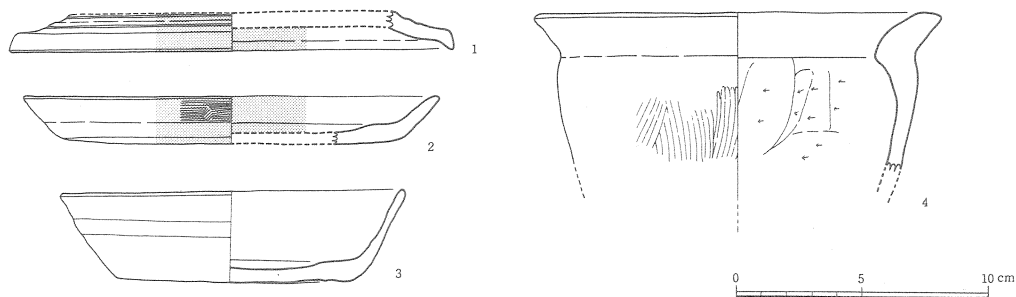
第59図 13号住居跡内出土土器実測図
