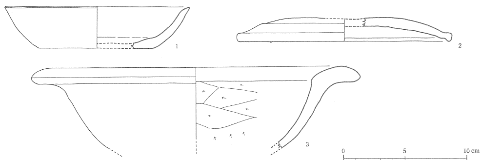
第63図 16号住居跡内出土土器実測図
