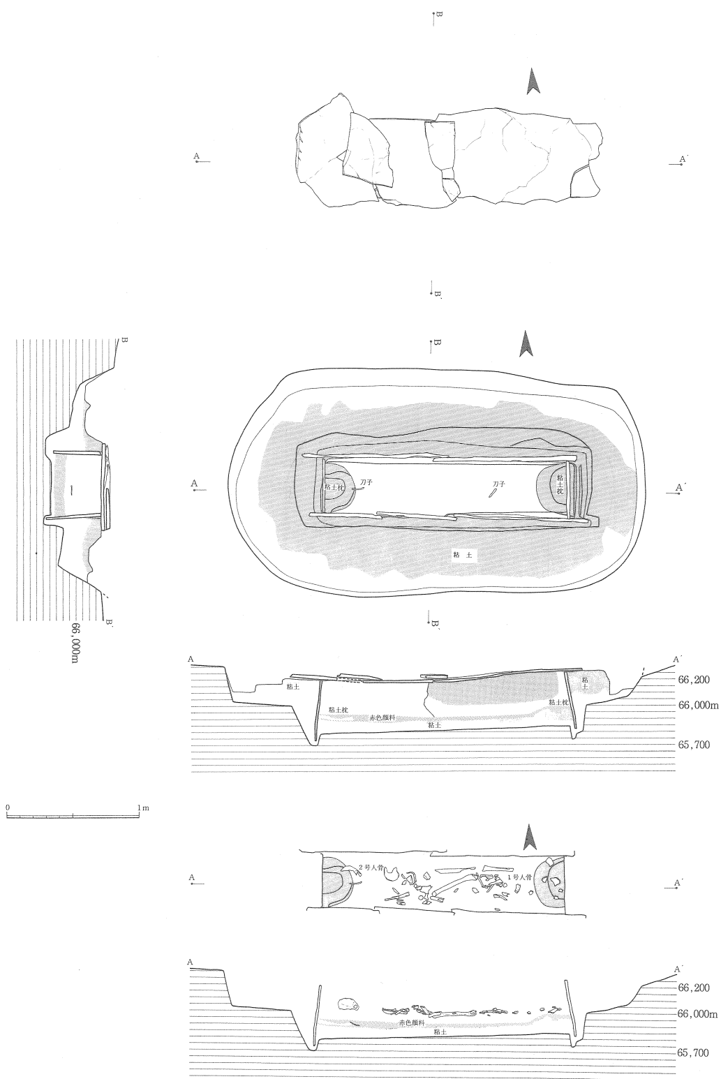
第32図 7号方形周溝墓主体部石棺及び石棺内人骨出土状態実測図
