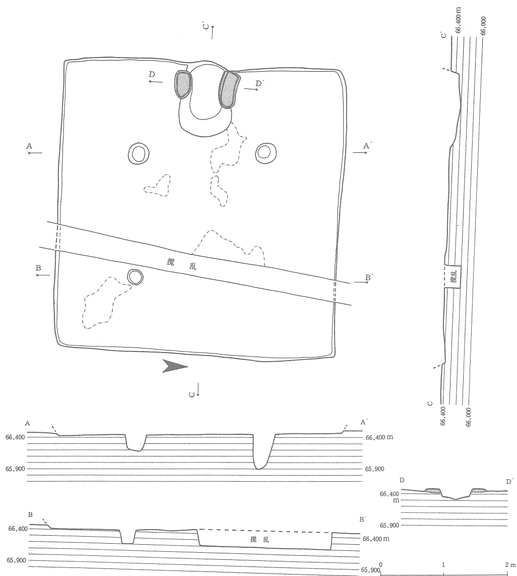
第102図 50号住居跡実測図
