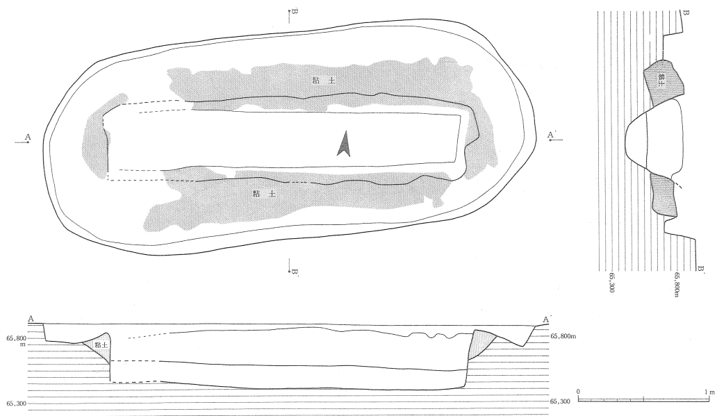
第7図 1号方形周溝墓主体部実測図
