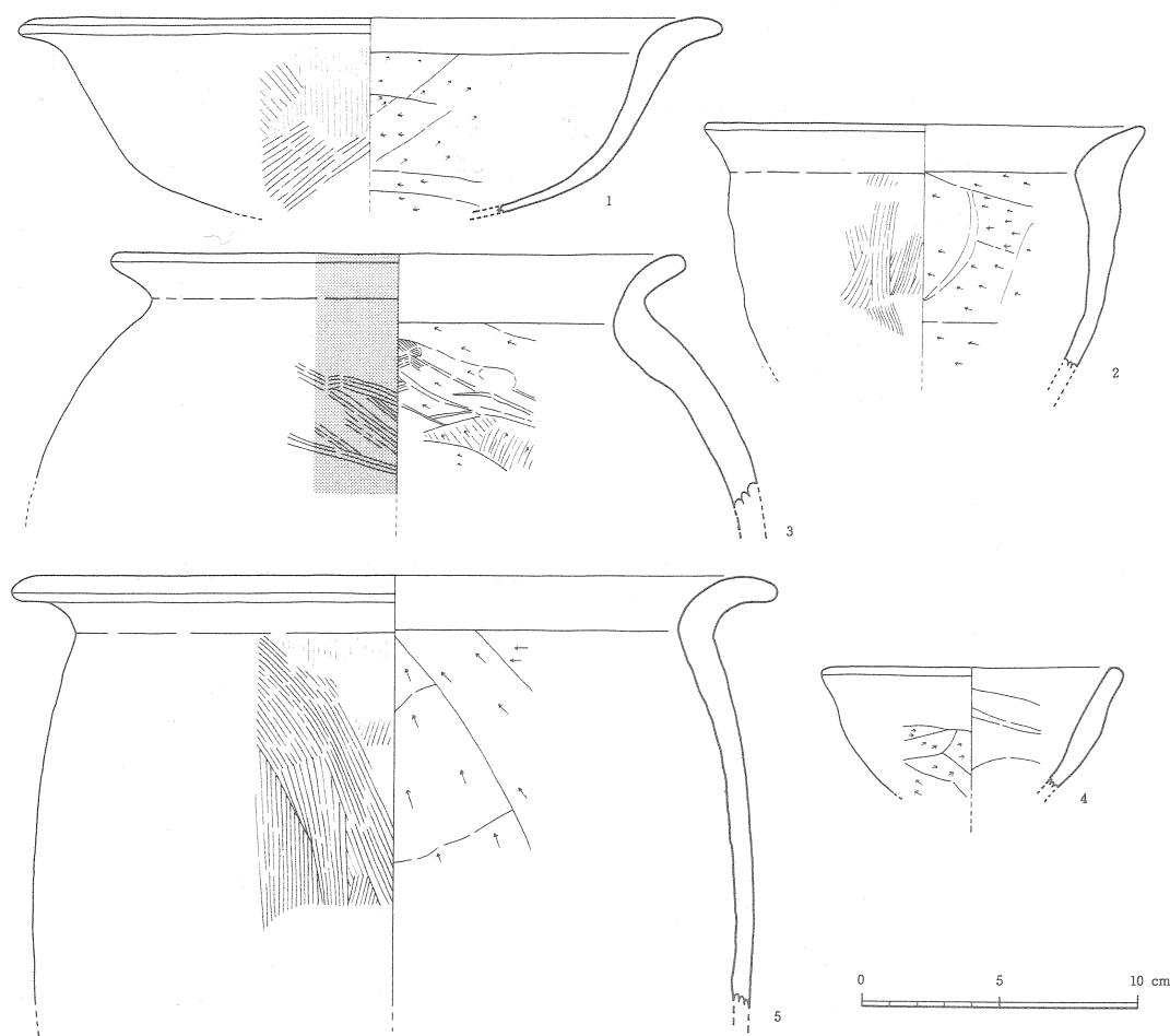
第87図 37号住居跡内出土土器実測図
