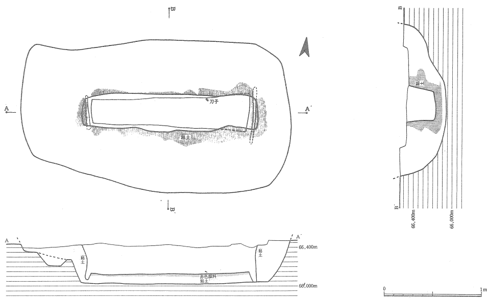
第21図 4号方形周溝墓主体部実測図
