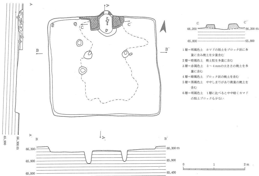
第108図 54号住居跡実測図
