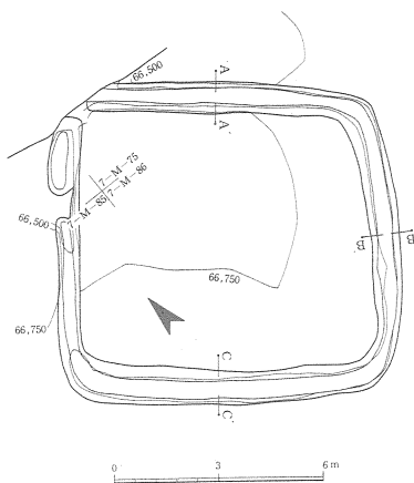
第38図 10号方形周溝墓測量図及び周溝土層断面図
