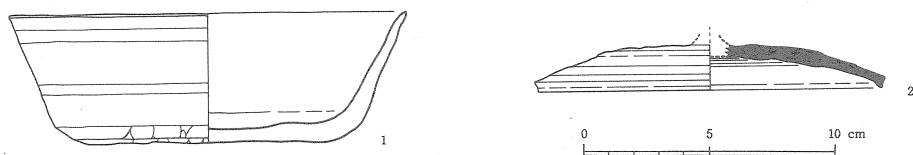
第97図 47号住居跡内出土土器実測図
