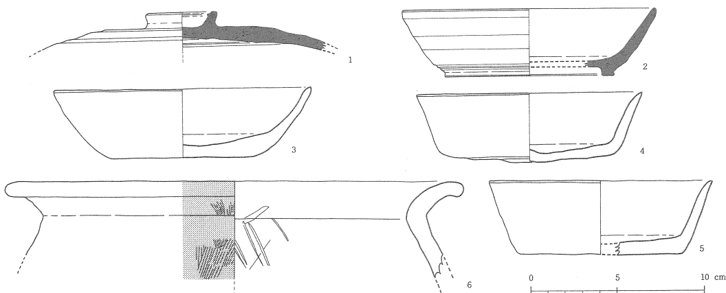
第90図 40号住居跡内出土土器実測図
