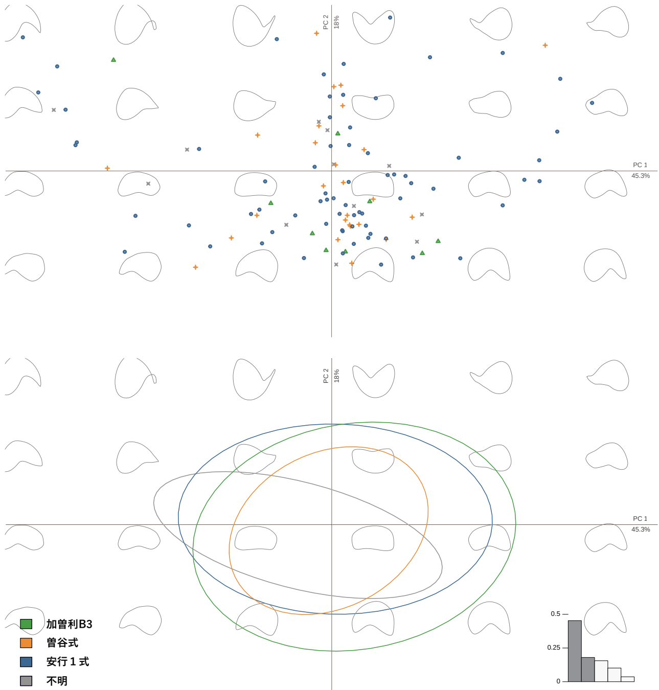
第4図 PC1, 2 の散布図 (上) と信頼楕円 (下)
