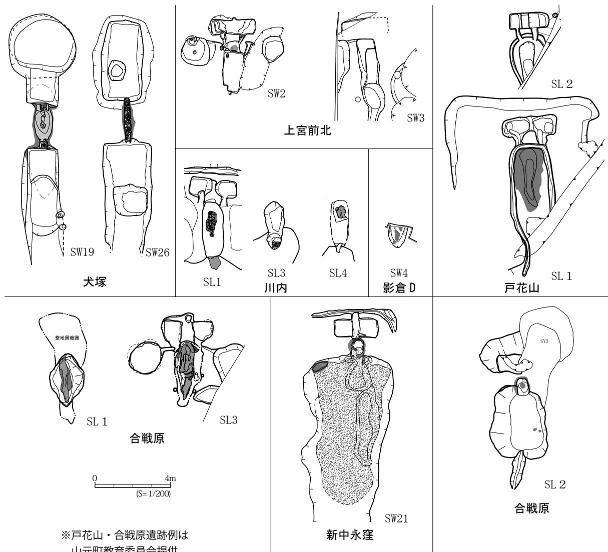
第5図 製鉄遺構集成 (文献17・18・23・24・25から作成)
