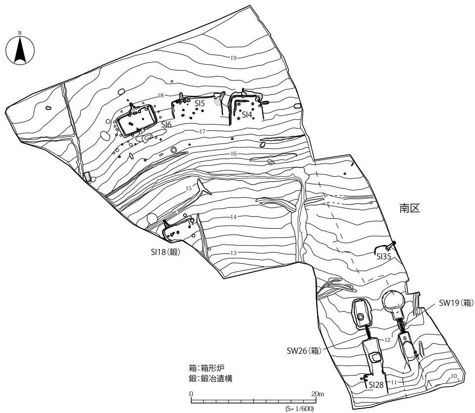
第2図 犬塚遺跡遺構配置図 (文献18)
