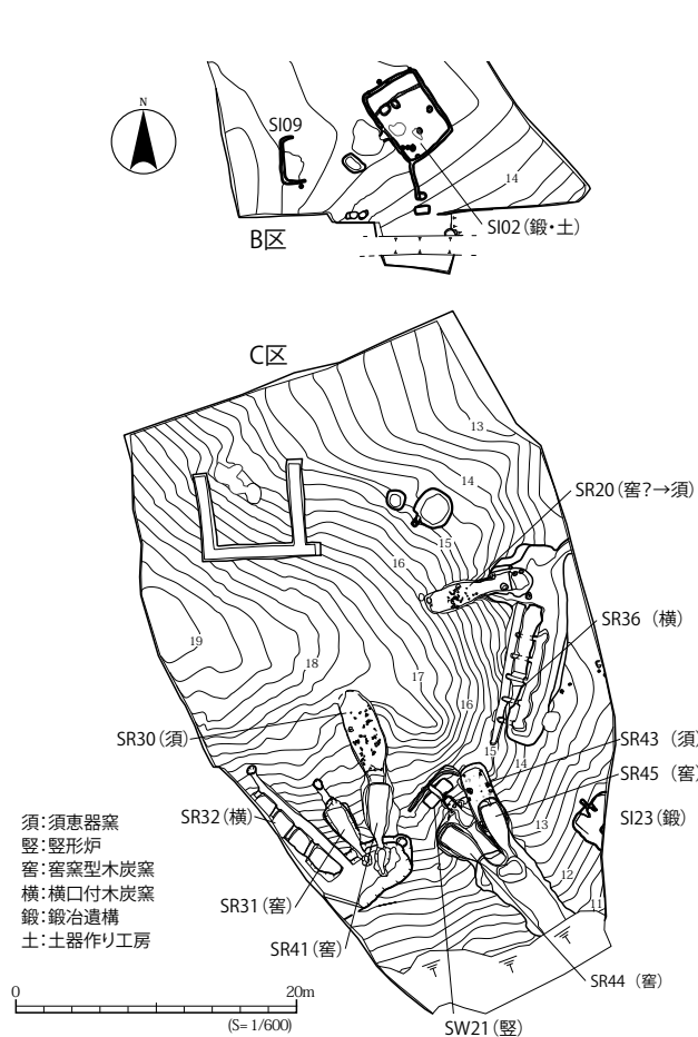
第3図 新中永窪遺跡遺構配置図 (文献18)
