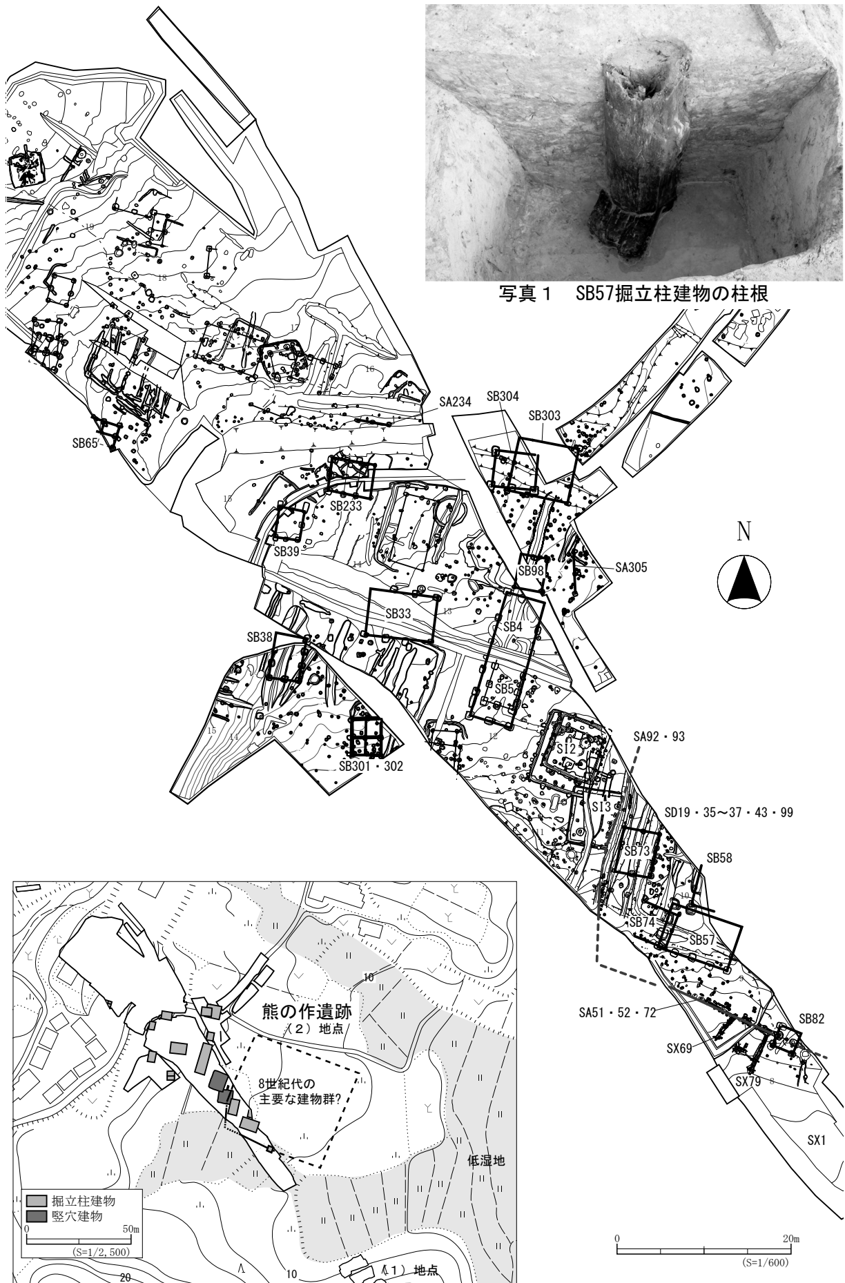
第2図 熊の作遺跡の主要な古代遺構配置 (宮城県 2016、山元町 2018 より作成)
