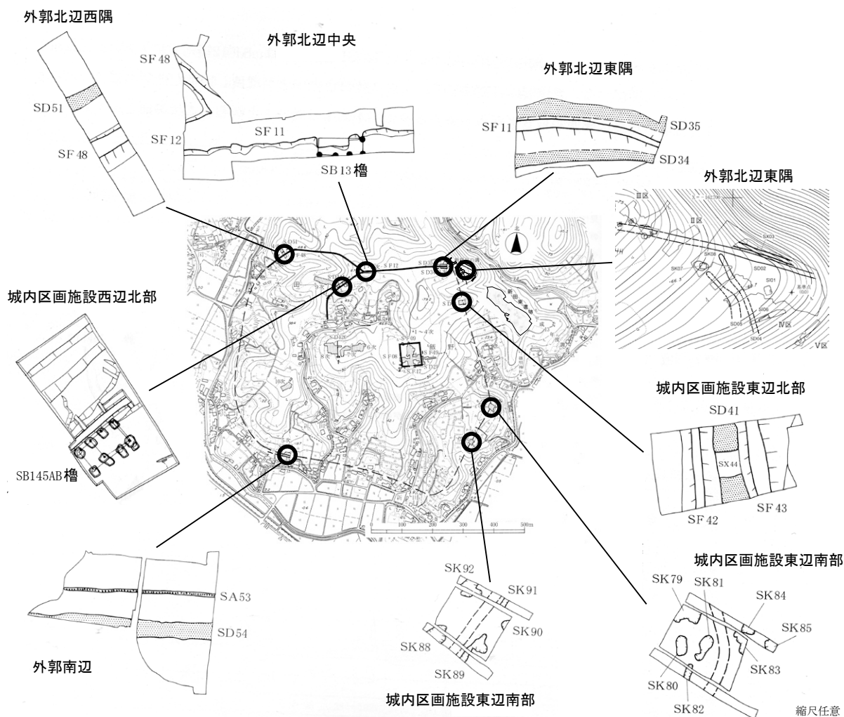
第3図 区画施設の平面図 (多賀城研 2001・2002・2004、宮城県 2003・2006 を改変)
