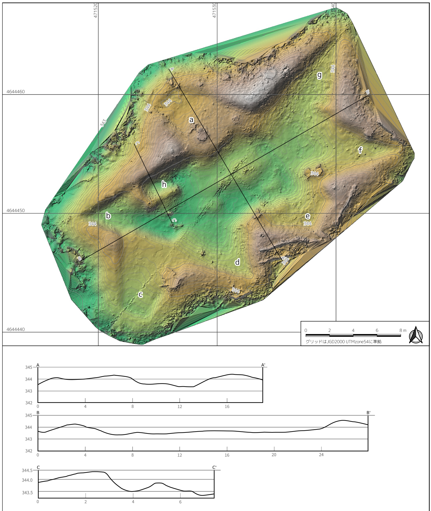
図 2.8 七飯町峠下台場測量図
