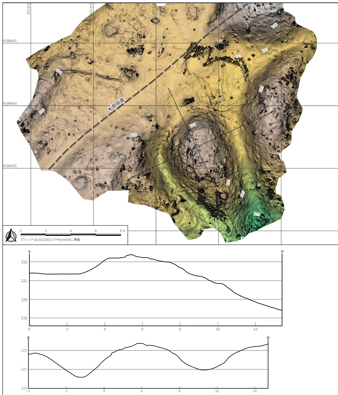
図 2.5 福島町茶屋峠台場測量図
