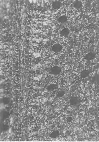
横断面 ————— : 0.4mm
