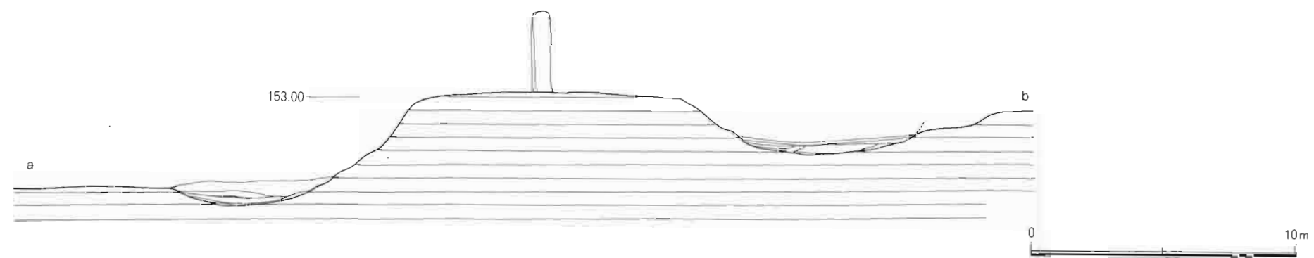
牧原千人塚測量図（1/200）
