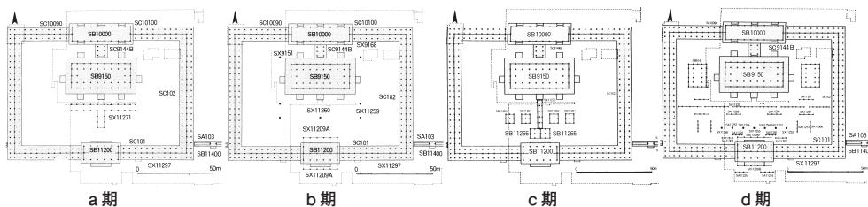
図2 第二次大極殿院地区Ⅱ期儀式遺構 『平城宮発掘調査報告XIV』、寺崎・金子案
