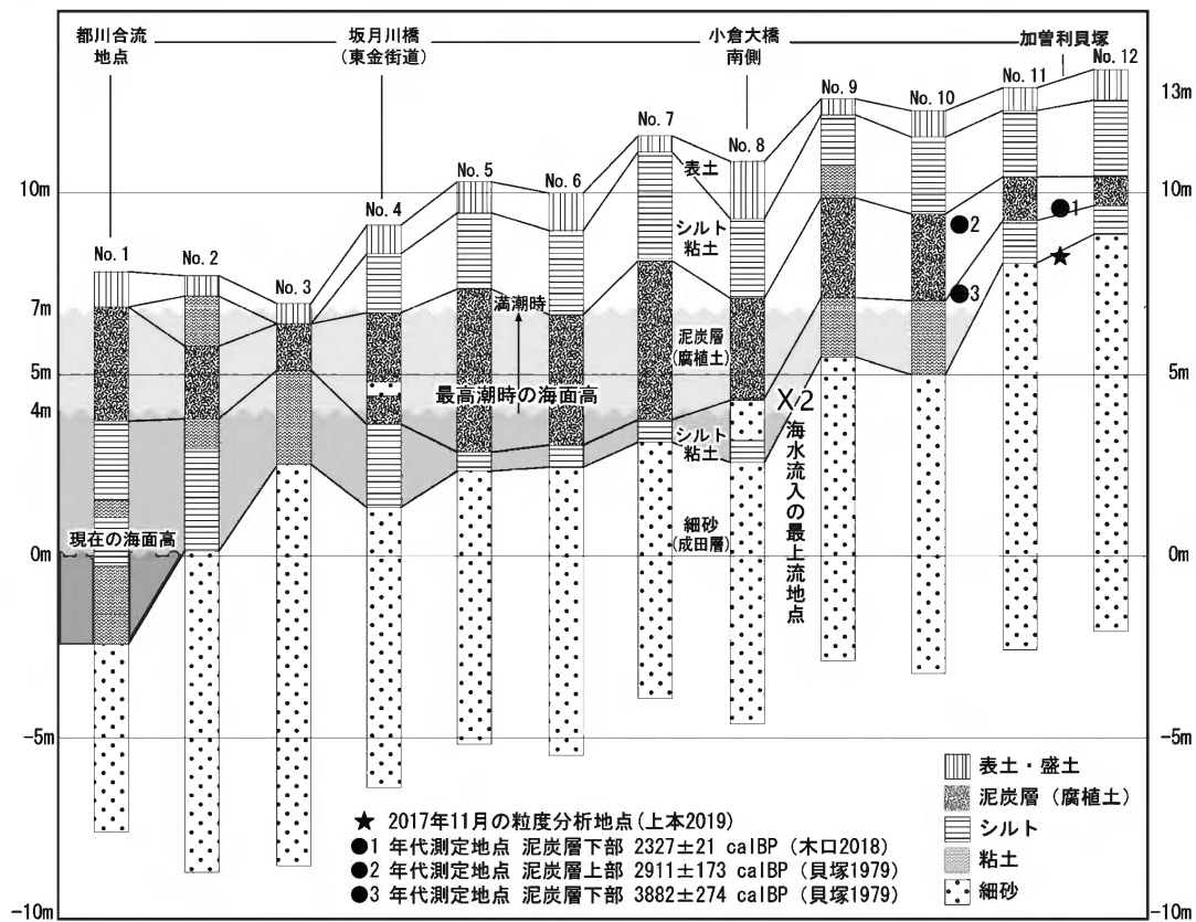
図3 坂月川の模式化柱状図
