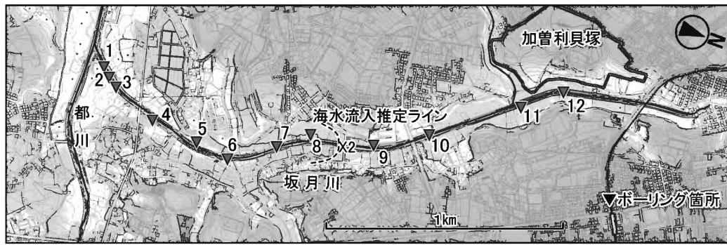
図2 坂月川ボーリング調査地点位置図
