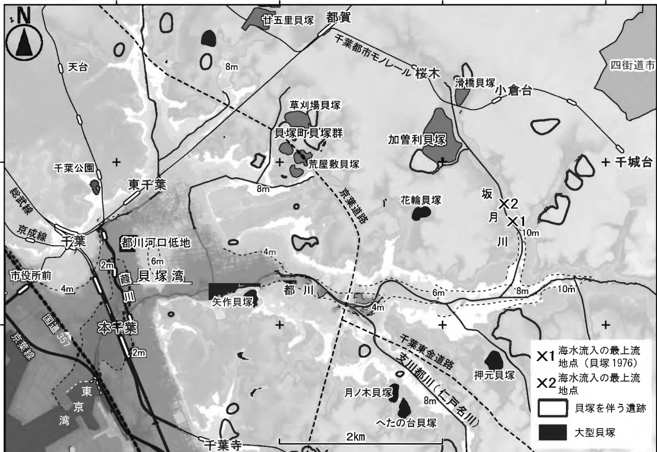
図1 都川流域と貝塚分布（図中の数値は現在の標高値）
