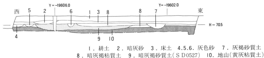
fig. 6 発掘区北壁東部土層図
