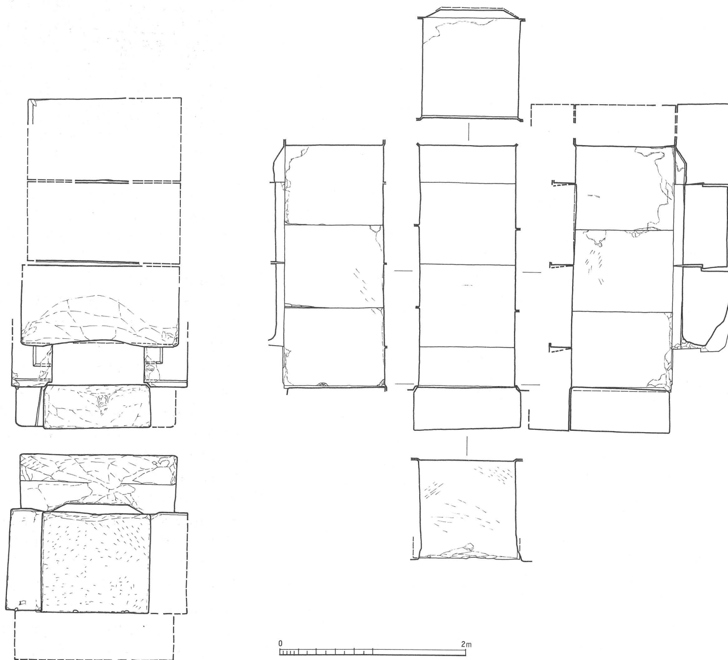
第 9 図 石室実測図
