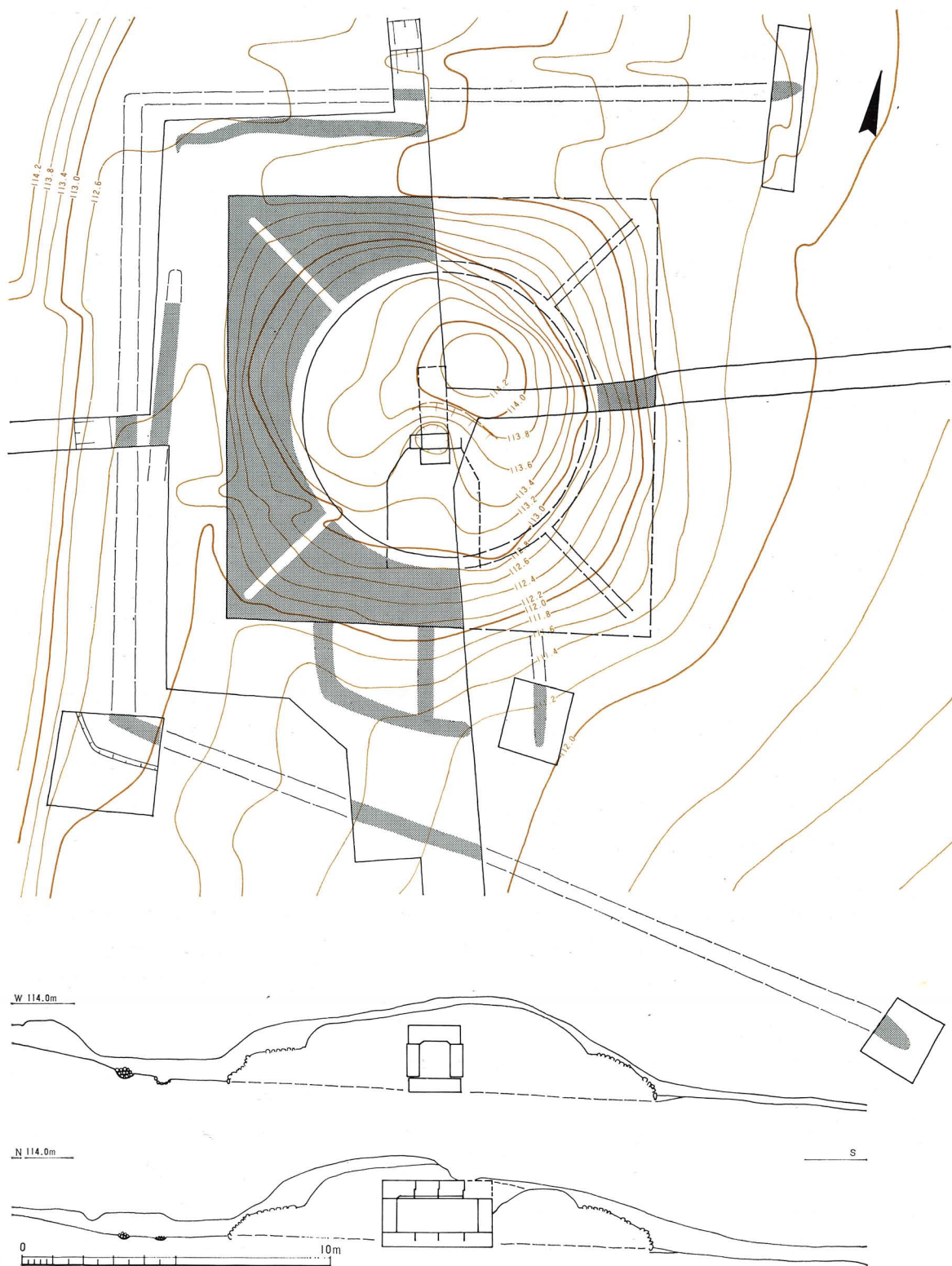
第5図 墳丘測量図
