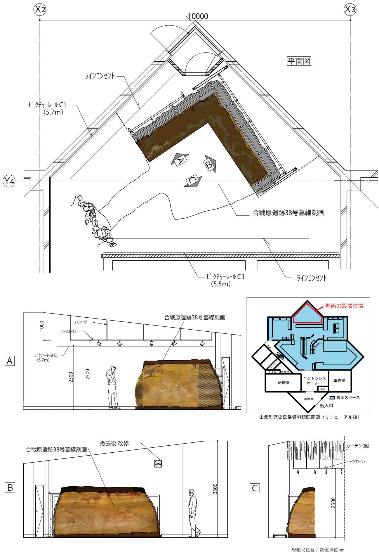
第100図 線刻壁画展示箇所の平面・立面図
