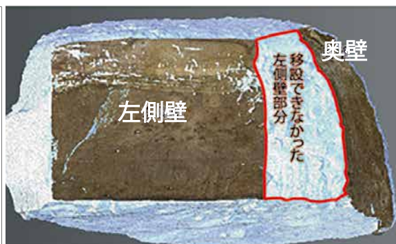
3. 【工程 10-(1)】 実物の 3 次元データと現地で取得した 3 次元データを重ね合わせた画像
