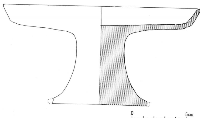
高杯実測図
