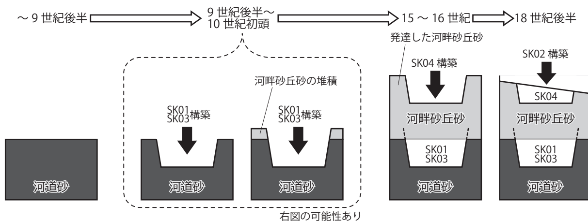
第62図 大林河畔砂丘形成と遺構構築の関係
