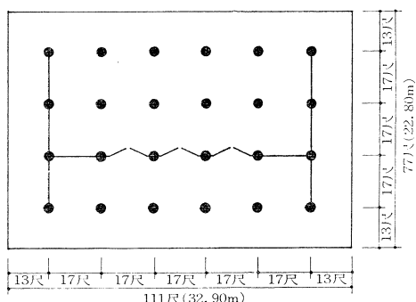
Fig 24 羅城門推定寸法 その1
