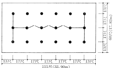
Fig 25 羅城門推定寸法 その2
