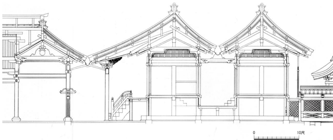
図2：石清水八幡宮本殿断面図
