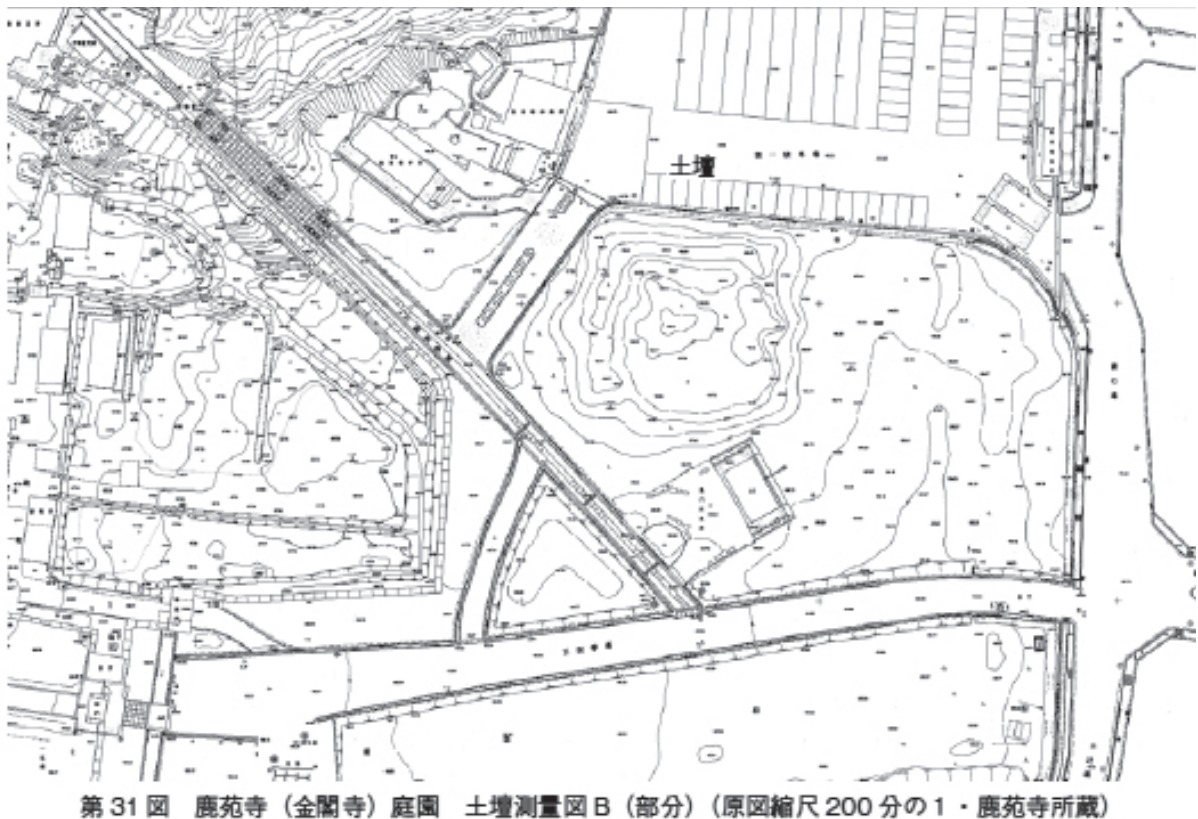
図5 昭和63年測量図B
