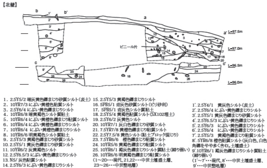
図8 土壇石垣部盛土断面図
