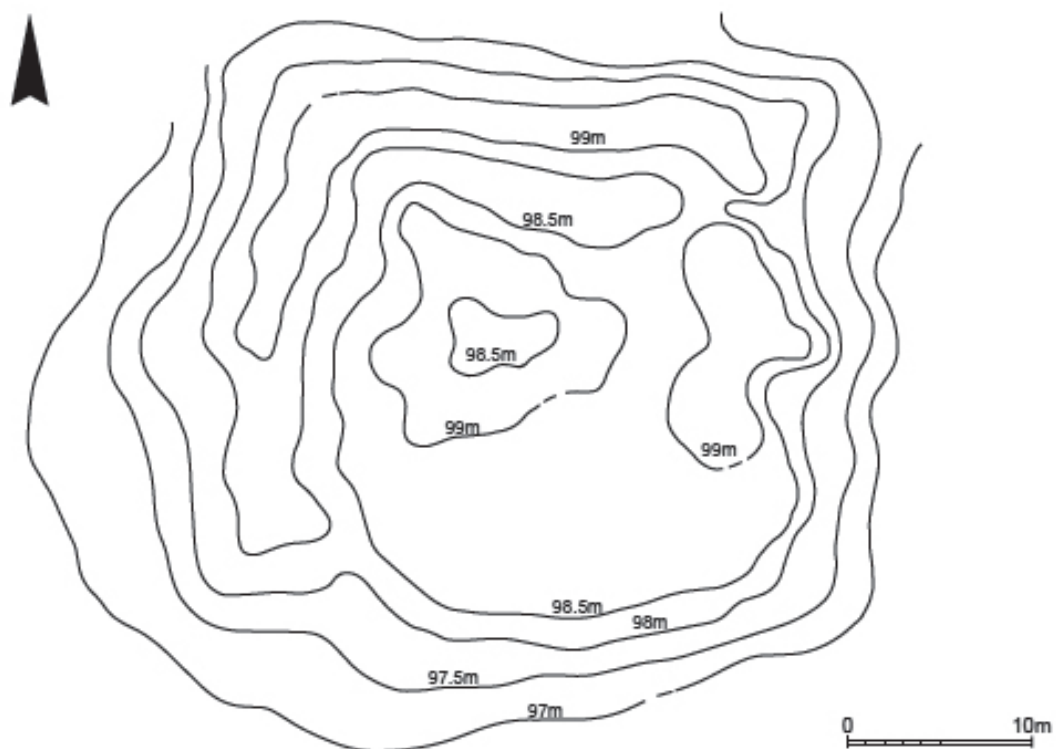
第 51 図 測量図 B 土壇部分 (S=1/400)
