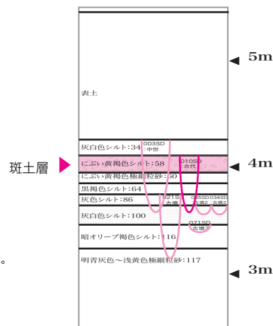
図5 12Fa区西壁北側基本層序模式図
