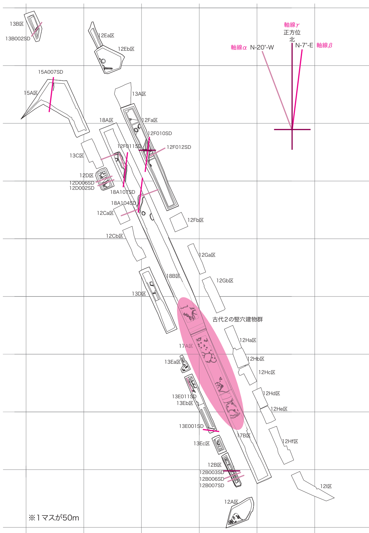
図6 北丹波・東流遺跡古代遺構全体図 S = 1:1000
