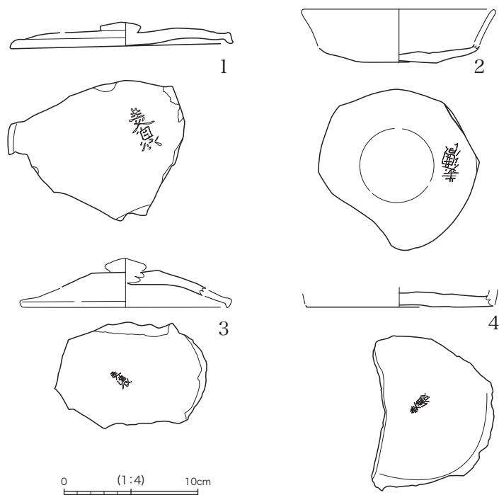
図8 江崎武氏旧蔵「美濃」施印須恵器実測図
