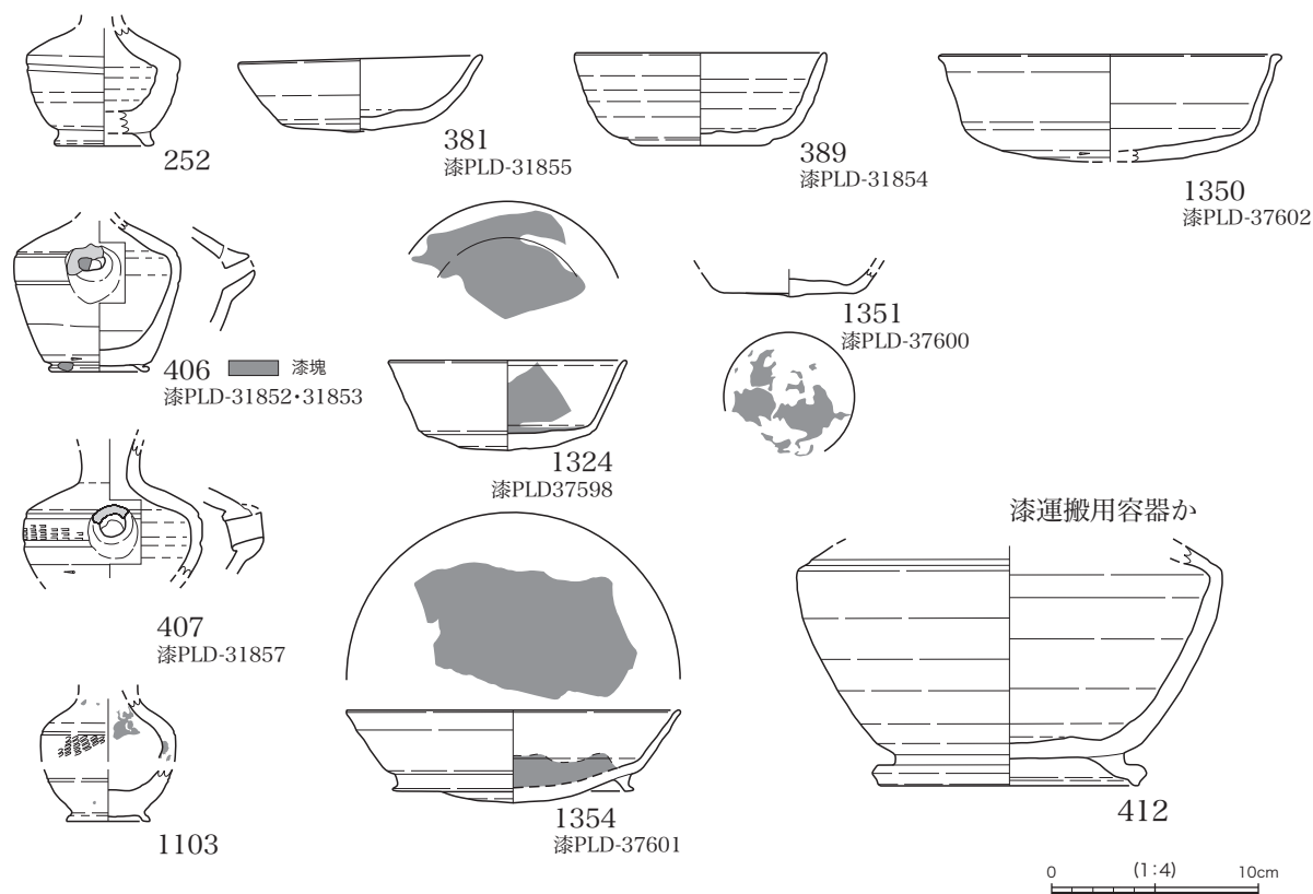
図10 北丹波・東流遺跡出土漆付着須恵器実測図
