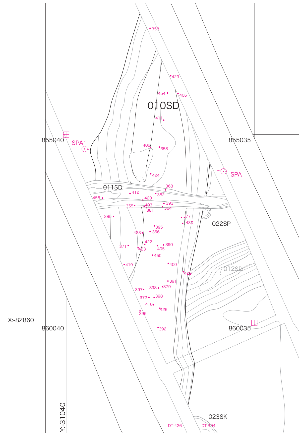
図2 12Fa区 010SD 遺物出土状態平面図 (S=1/50)
