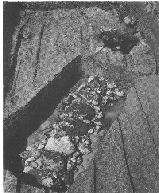
石組暗渠 SD2430（第58—20次調査）
