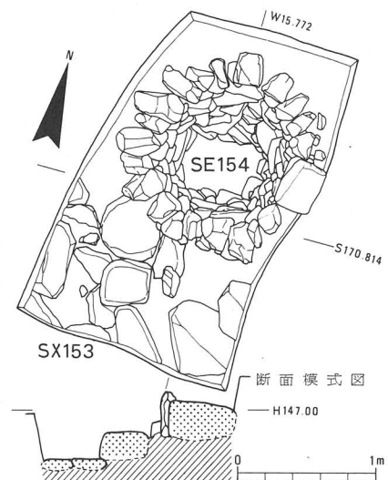
第31図 調査遺構配置図 (1:50)
