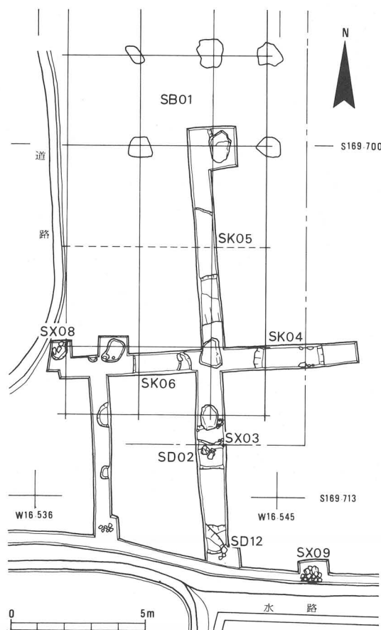
第23図 A調査地遺構配置図(1:200)
