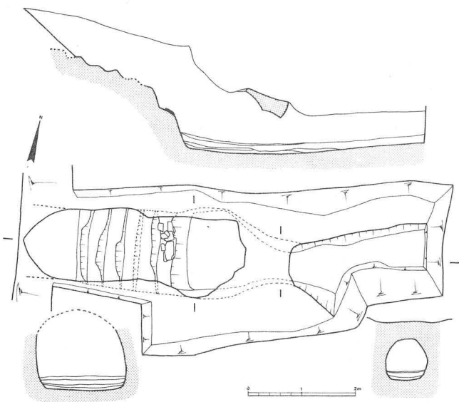
瓦窯実測図 (1/100)
