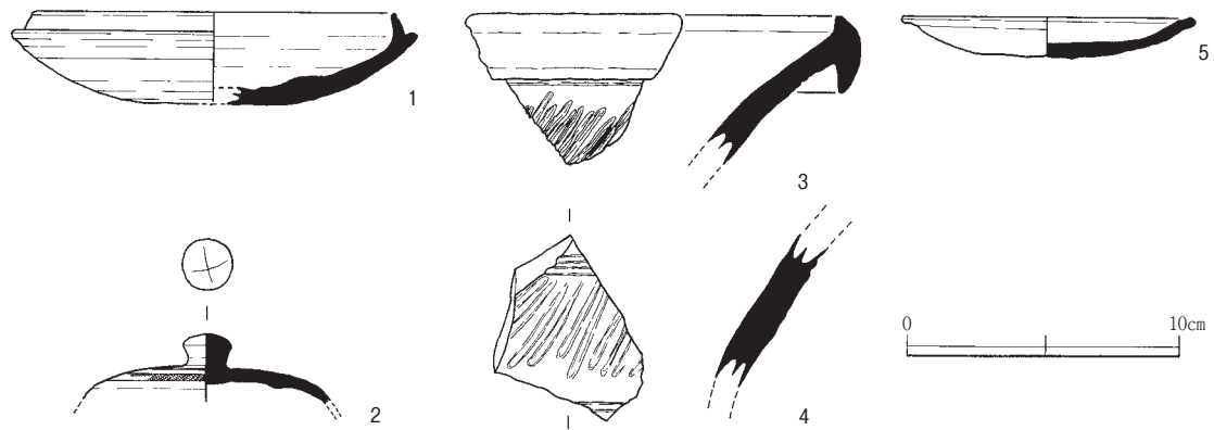
図11 土器実測図 1 : 3
