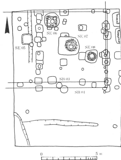
第16図 東僧房北方調査遺構図
