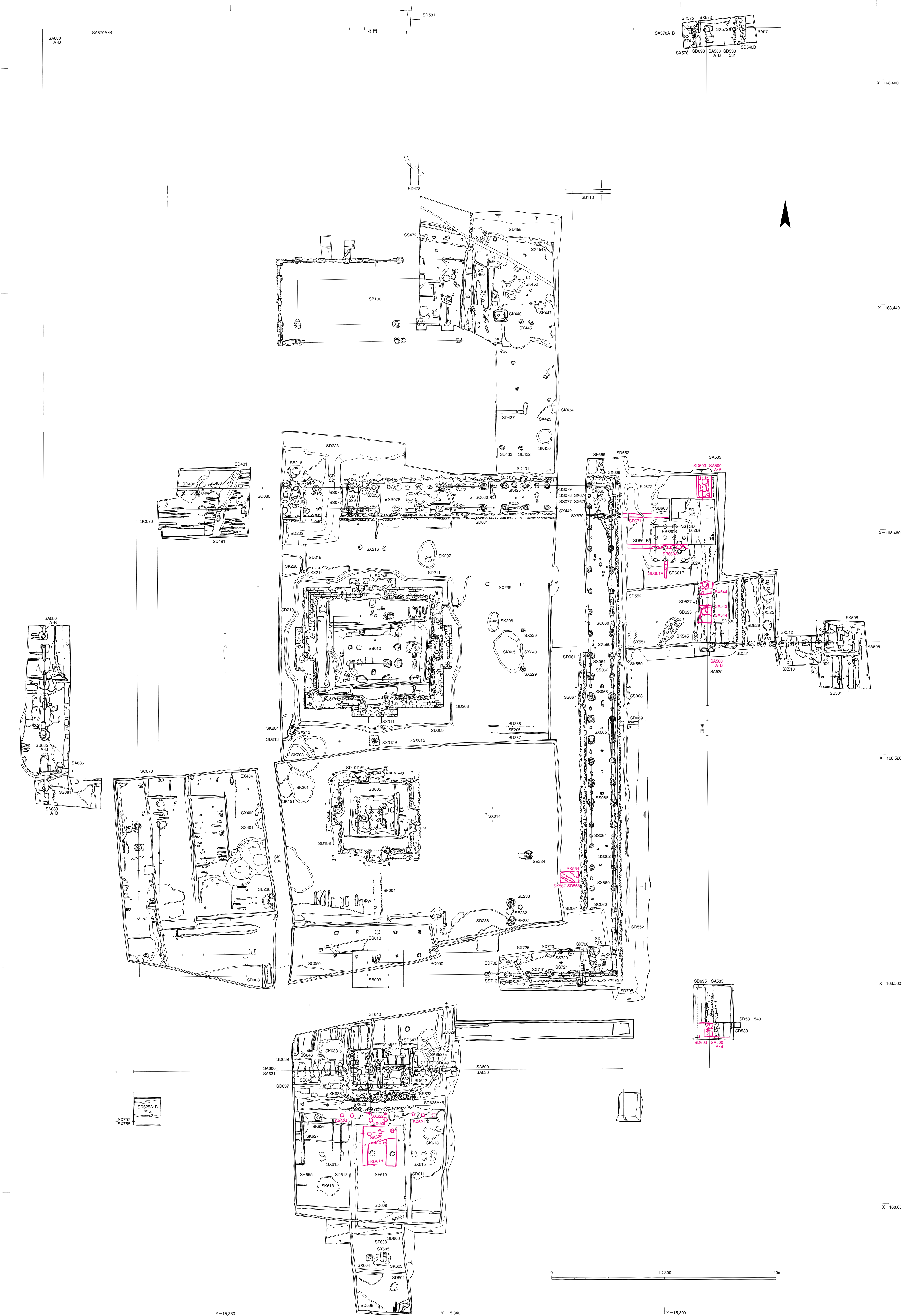
付図 1 山田寺遺構全図
