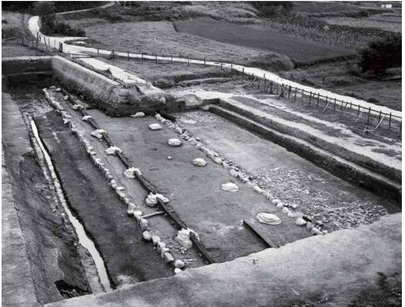
1 完掘状況 北東から
