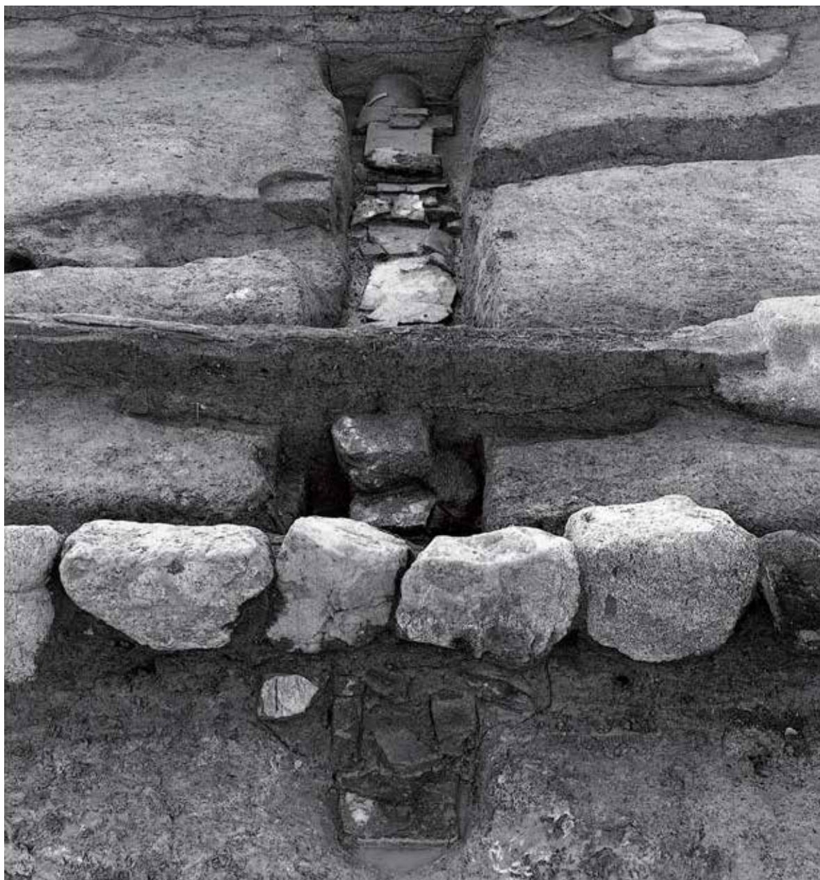
1 暗渠 SX670 東から
