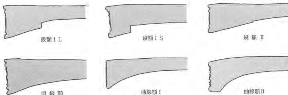
Fig. 34 軒平瓦の顎形態の分類
