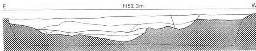
Fig. 31 SK 2001 断面図
