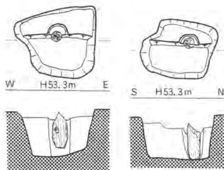
Fig. 27 SB 2065 の柱根
