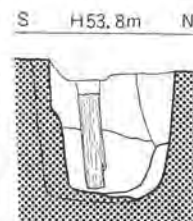
Fig. 25 SB 1830の柱根
