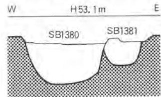
Fig. 23 SB 1380・1381 の重複
