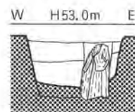
Fig. 33 SB 1326の柱根
