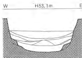
Fig. 28 SK 1348 断面図
