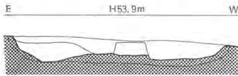
Fig. 30 SK 1943 断面図
