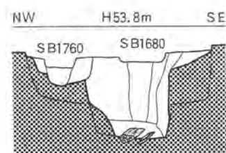
Fig. 14 SB 1680 の礎盤
