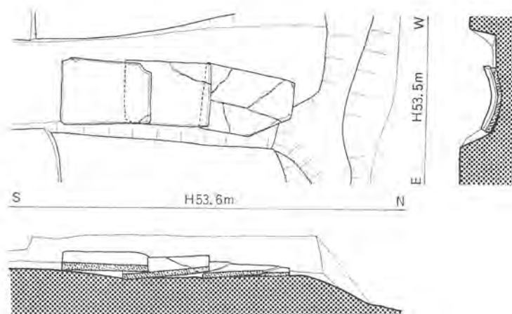
Fig. 21 SX 1489 断面図 (1:20)
