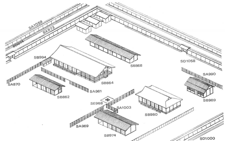
fig. 36 十五坪A 1期建物復原図
