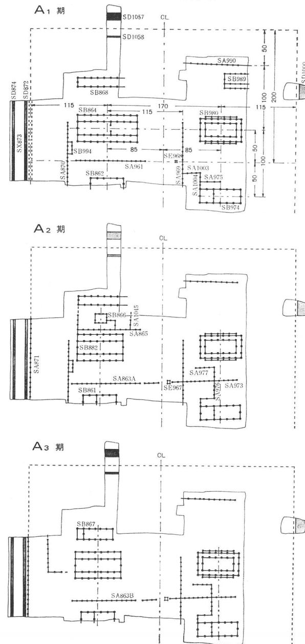
fig. 8 十五坪建物配置変遷図 I 15
