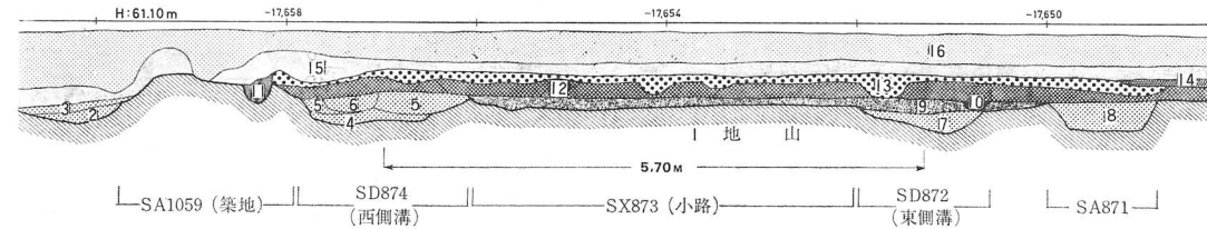
fig. 7 SX873断面図
