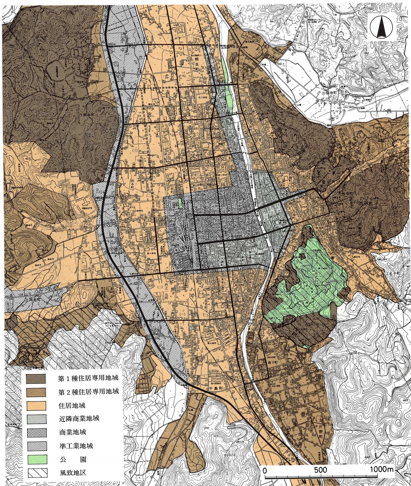
8 道路・都市計画図
