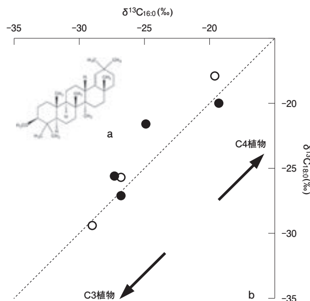
図35 ミリアシンの化学構造式 (a) および個別脂肪酸 (パルミチン酸、ステアリン酸) の安定炭素同位体比 (b) (●はミリアシンが検出された試料、○は検出されなかった試料を示す。)
