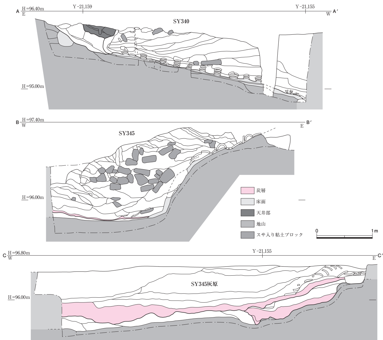
図243 瓦窯SY340・345土層図・断面図 1:40
