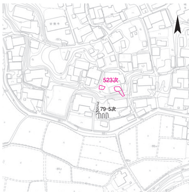
図238 第523次調査区位置図 1:2500
