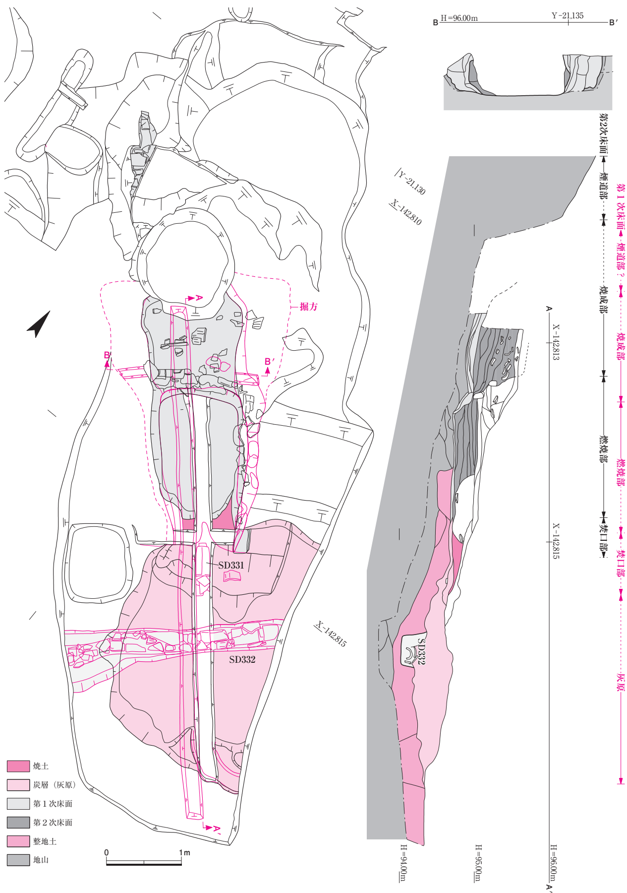
図241 瓦窯SY330遺構図・断面図 1:50
