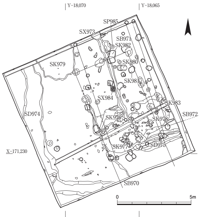
図176 第180次調査B区遺構図 1 : 150
