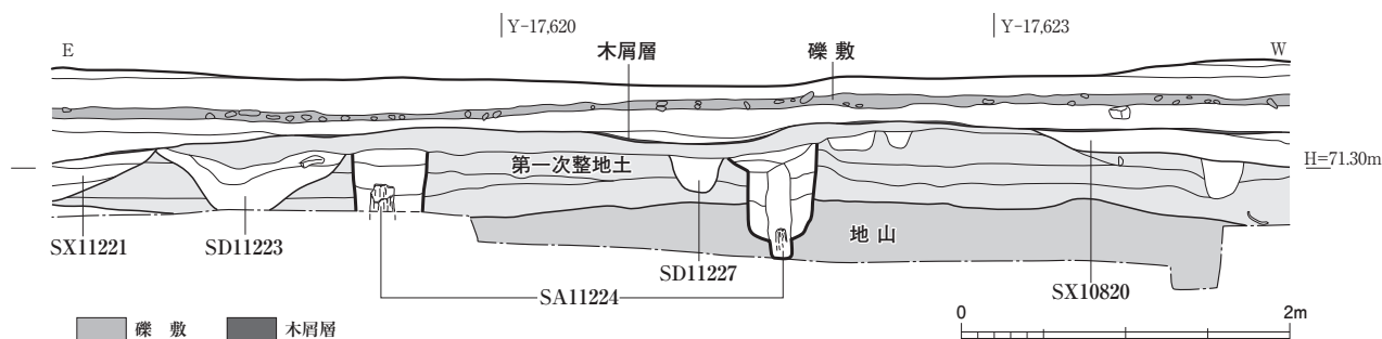
図Ⅱ-6 調査区南壁土層図 1:50
