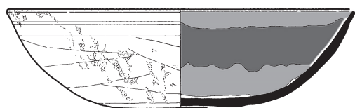
図I-70 平城京漆紙文書第8号土器実測図（1：2）
