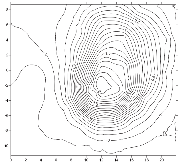
図 I-18 1号窯跡測量図
