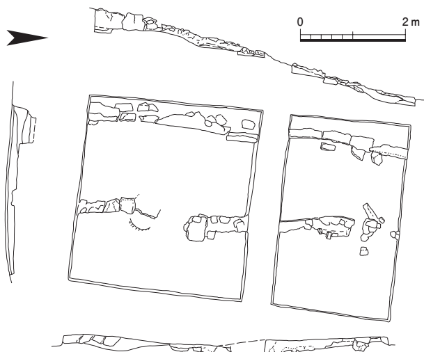
図 I-19 1号窯トレンチ平面図 1:20
