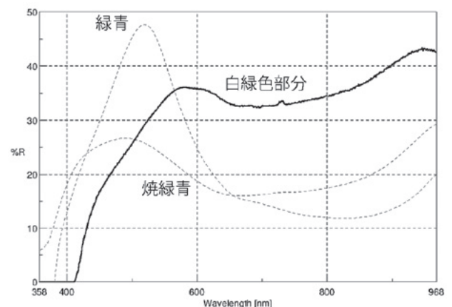
図106 裳階上支柱飾獣形彫刻 (347) の白緑色部の分光スペクトル
