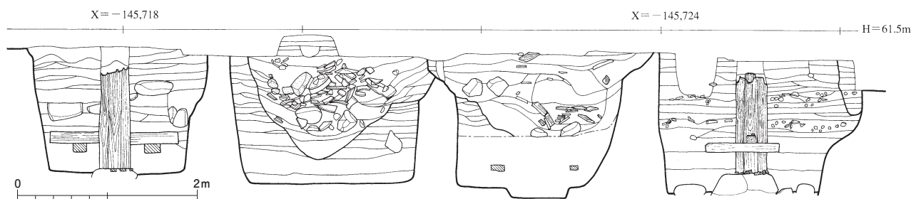
図77 平城宮東院庭園SB5880の東側柱穴列断面 1:60
