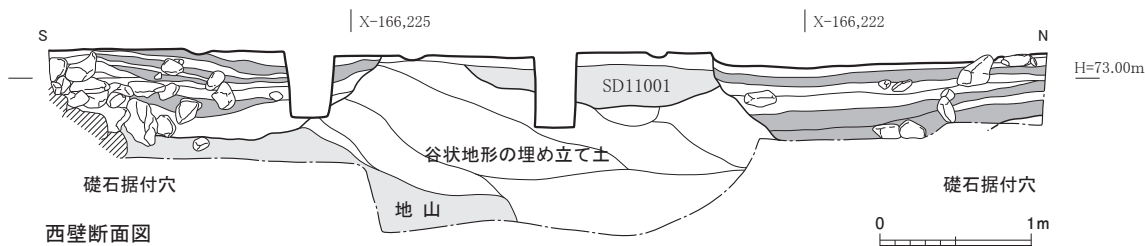
図76 藤原宮東面中門SB11000の礎石据付穴と版築 1:50
