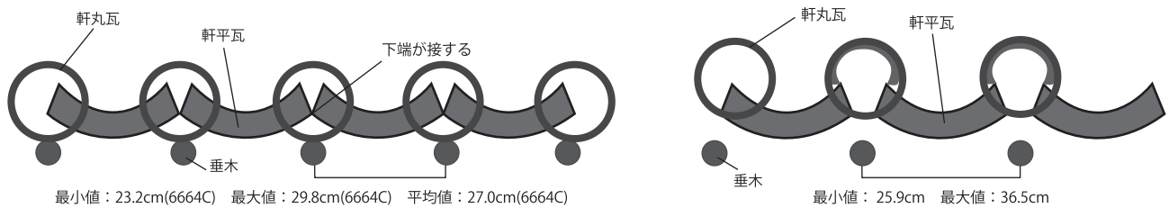
図67 瓦葺想定模式図（左：想定1、右：想定2）
