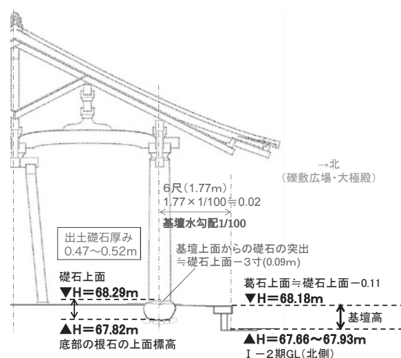
図64 南面回廊北側基壇断面模式図
