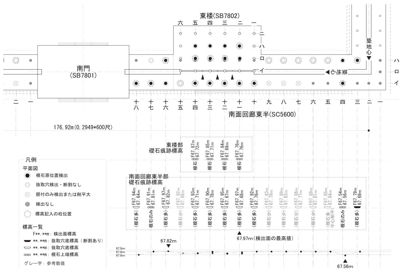
図63 Ⅰ-2期南面回廊礎石痕跡標高の模式図(南面回廊西半は省略)
