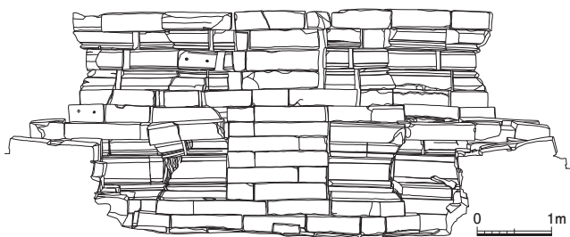
図13 南祠堂基壇内北立面図（中央祠堂南階段）
