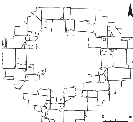
図11 上成基壇N16平面図
