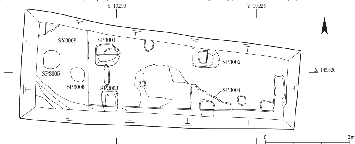
図238 第484次調査遺構平面図 1:80
