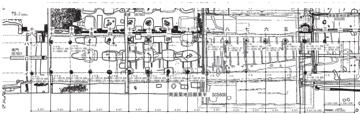
図89 南面築地回廊東半 SC5600 遺構図+想定平面模式図（I－1期）
