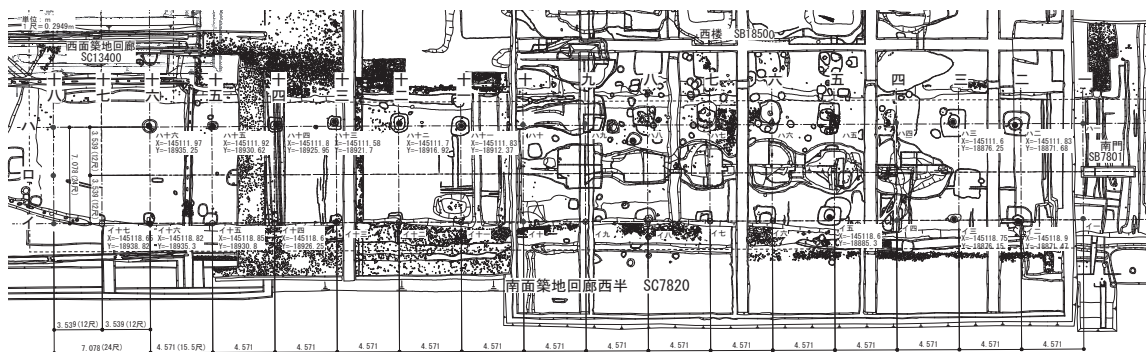
図90 南面築地回廊西半 SC7820 遺構図+想定平面模式図（I－1期）
