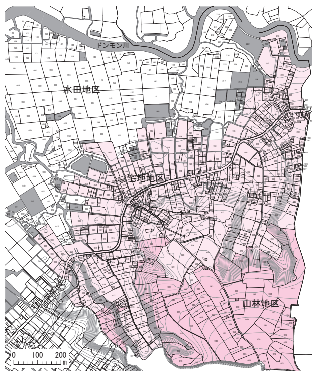
図37 フーホイ村フーミーⅡ集落の土地利用
