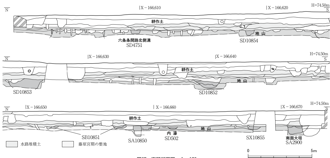
図67 東壁断面図 1 : 150
