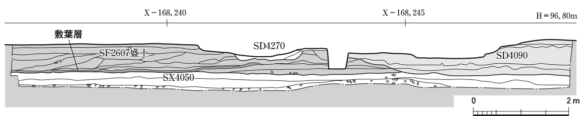
図118 SF2607断面図 1：80
